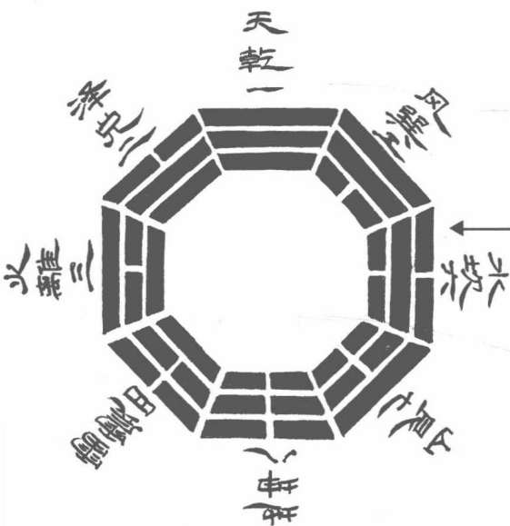
八卦图
