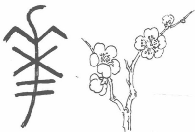
“华” 的古字
