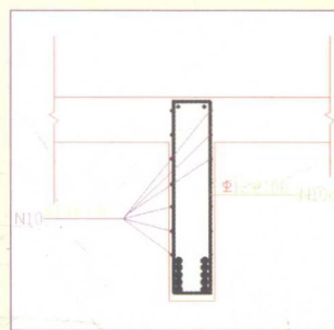
钢筋剖面
