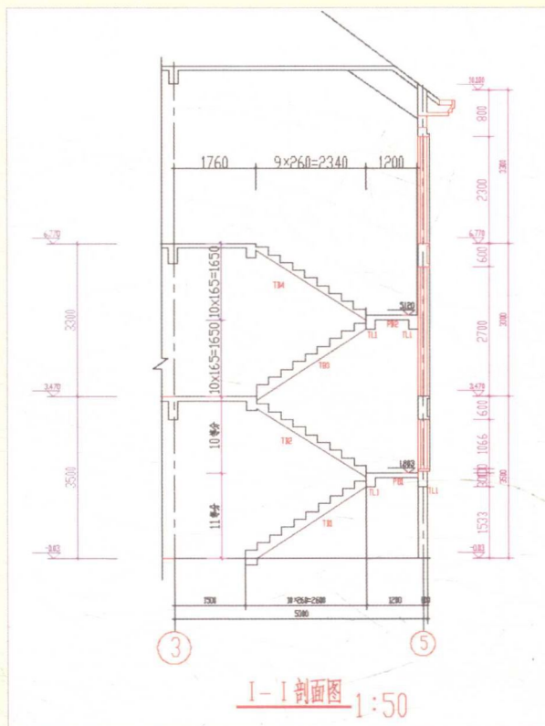
楼梯 1-1 剖面图
