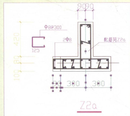
配筋绘制和标注
