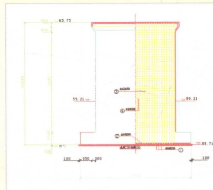
桥中墩剖面图绘制
