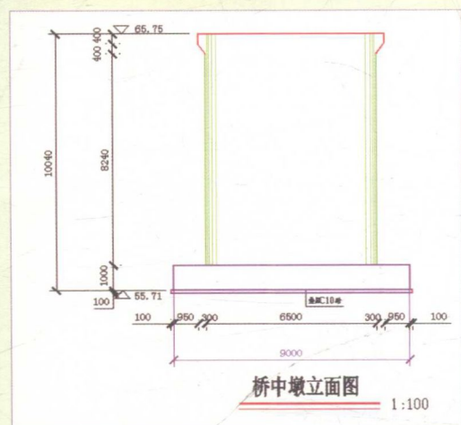
桥中墩立面图绘制
