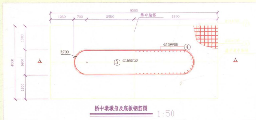
桥中墩墩身及底板钢筋图绘制
