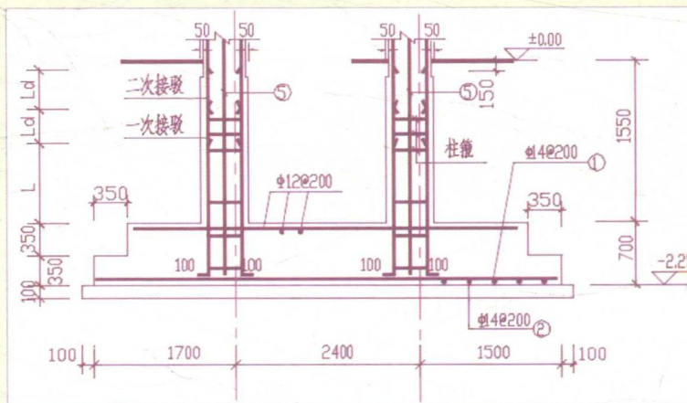
别墅基础详图绘制 (部分)
