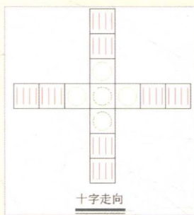
十字走向交叉口盲道
