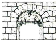
6. 将缺口做整齐,在缺口上方摆起楔形的石块(拱石)使之互相支撑,用一个木架将其稳住,拱做好后再把木架拿走。
