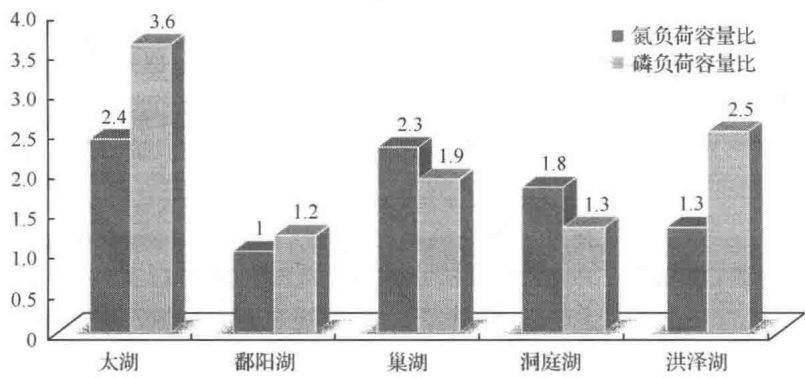
图 1-1 重点湖泊负荷容量比
