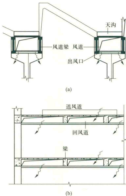
图 0.3.1 通风道与结构构件的合理结合
