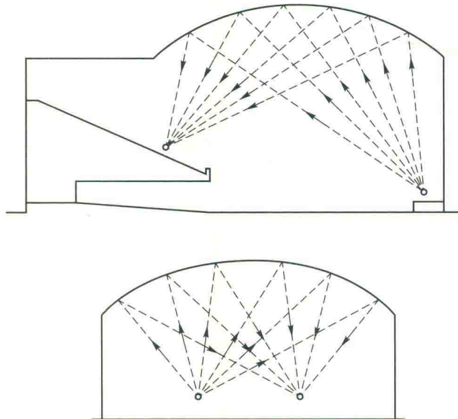
图 0.1.3 拱形天棚的声音聚焦现象
