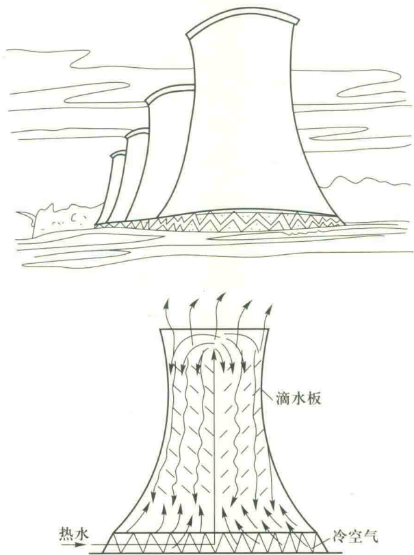
图 0.1.2 双曲抛物面冷却塔
