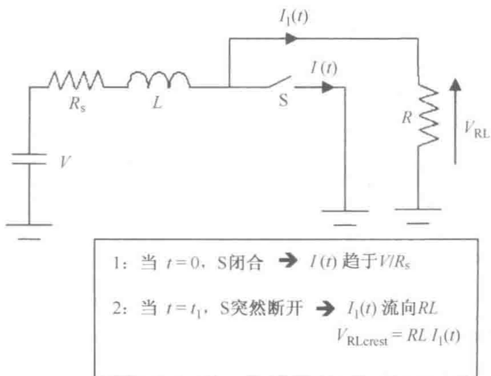
图4 电压型电感储能系统（其基本原理是在电感中产生电流，并迫使电流在特定时刻流经一个电阻，该系统需要分段能力强的开关）
