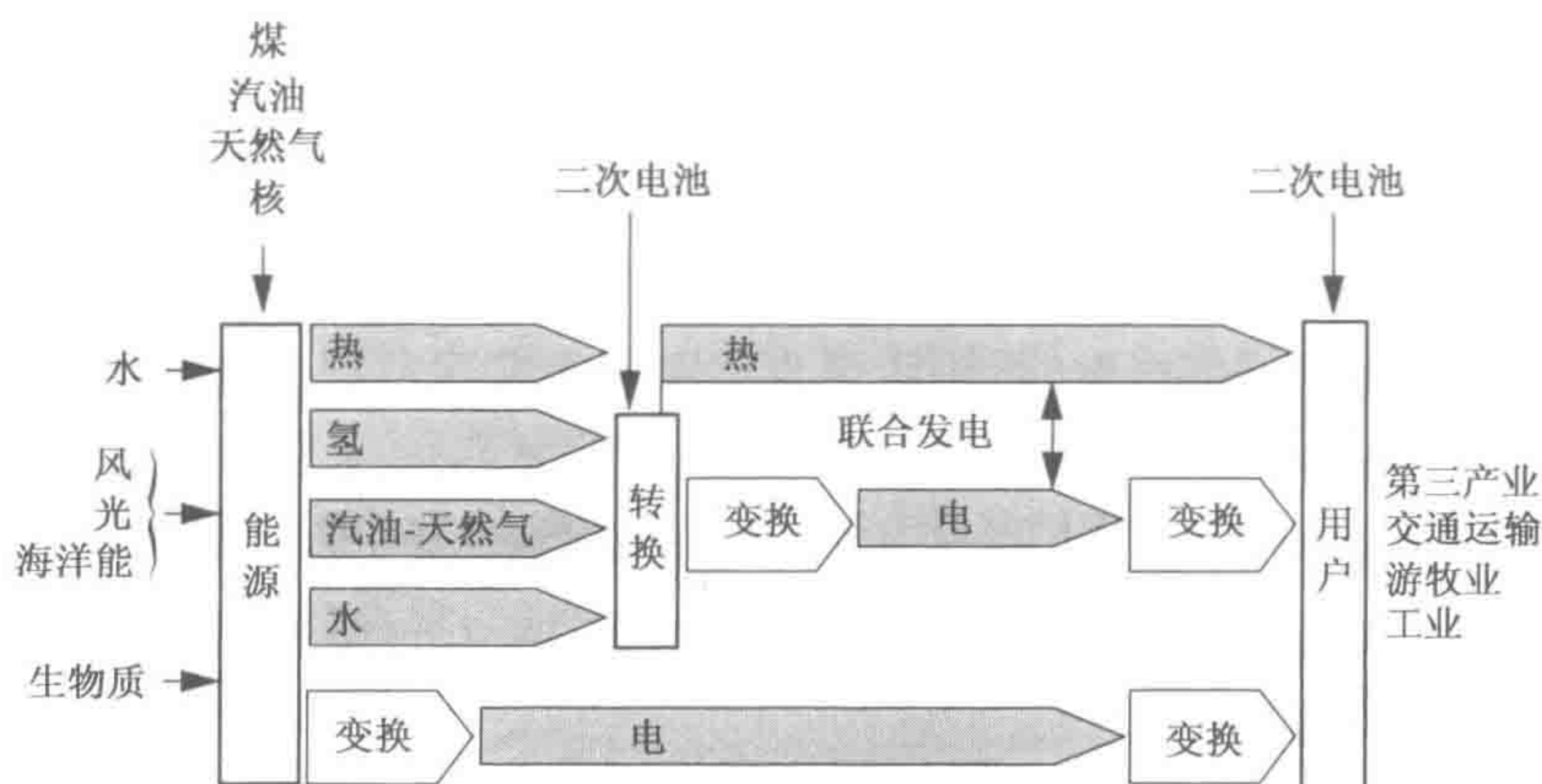
图3 储能装置的运行原理
