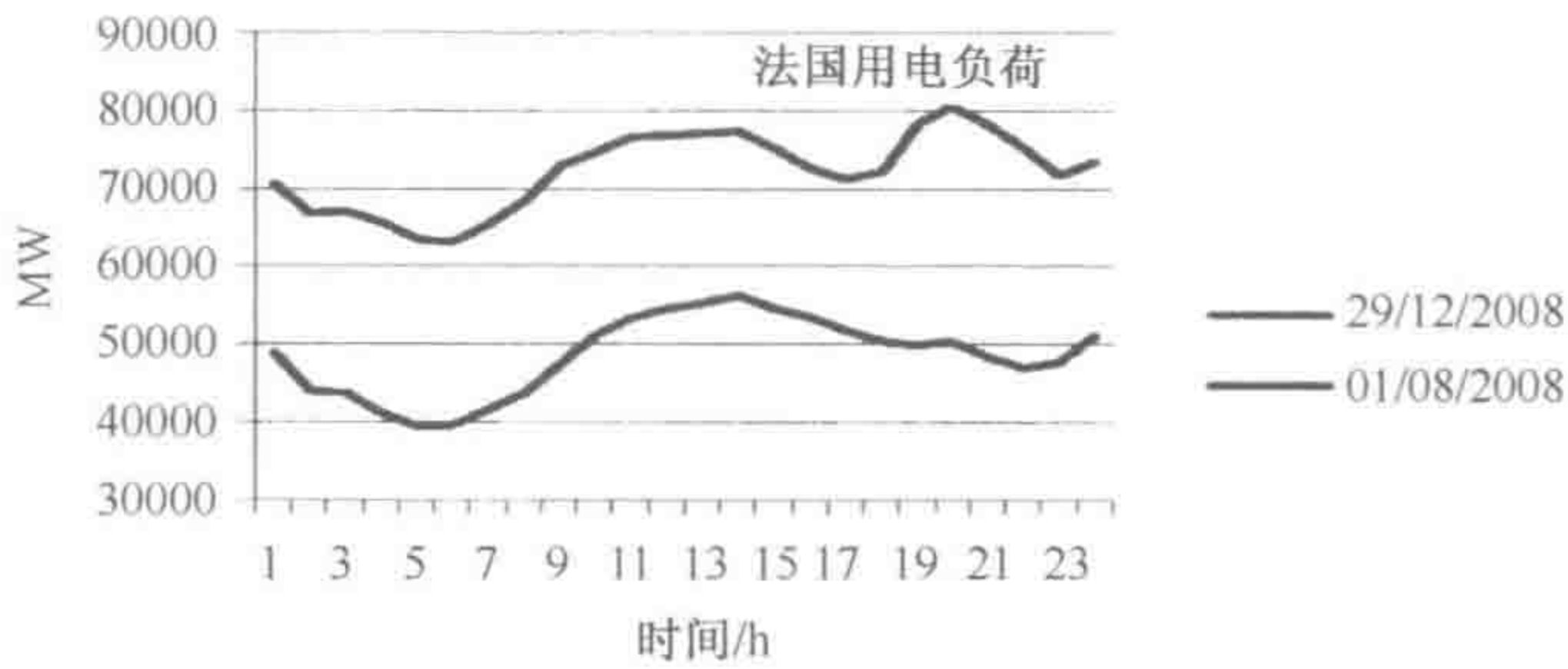
图6 法国的用电情况 (资料来源: RTE)
