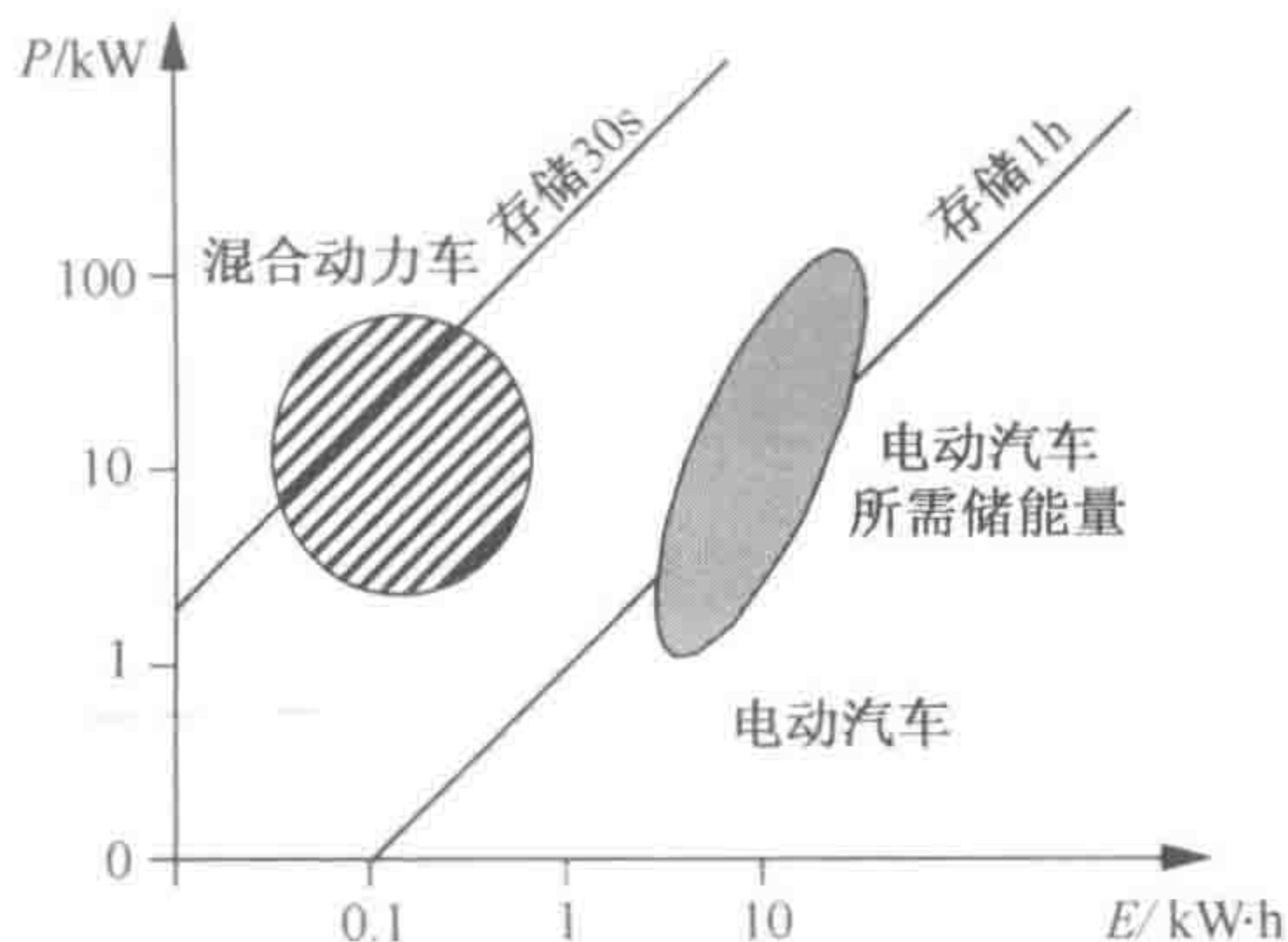
图2 电动汽车的储能需求（混合动力汽车关注储能所能提供的功率，而纯电动汽车则既关注功率也关注能量。对于混合动力汽车，所需的储能量约为 12\text{W}\cdot\text{h}/\text{kg} ，功率约为 500\text{W}/\text{kg} ，能够在 2s 内以 10\text{kW} 的功率提供 300\text{W}\cdot\text{h} 的能量，储能装置的寿命预期为 15 年）
