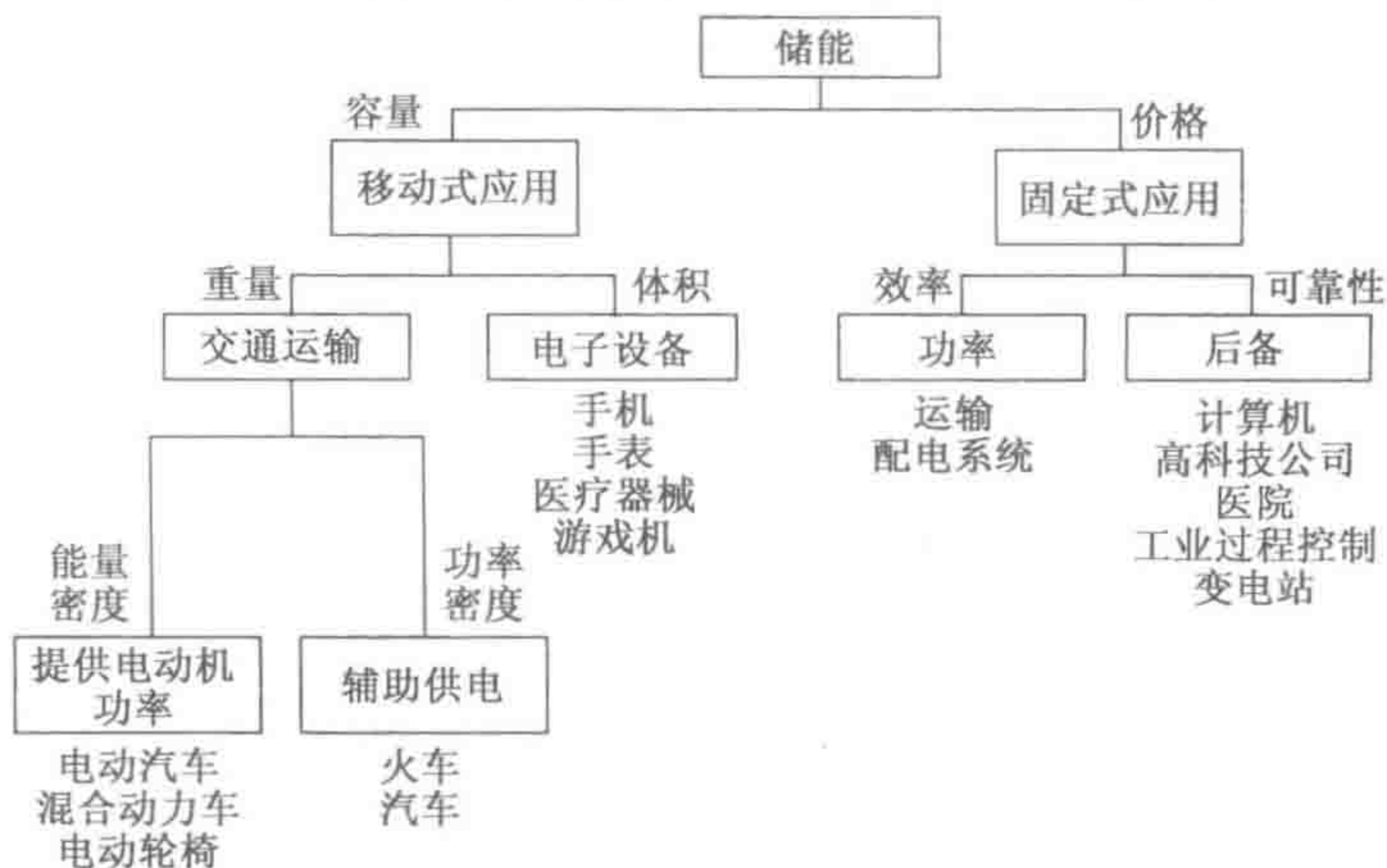
图 9 不同应用目标下储能的选择标准与约束条件
