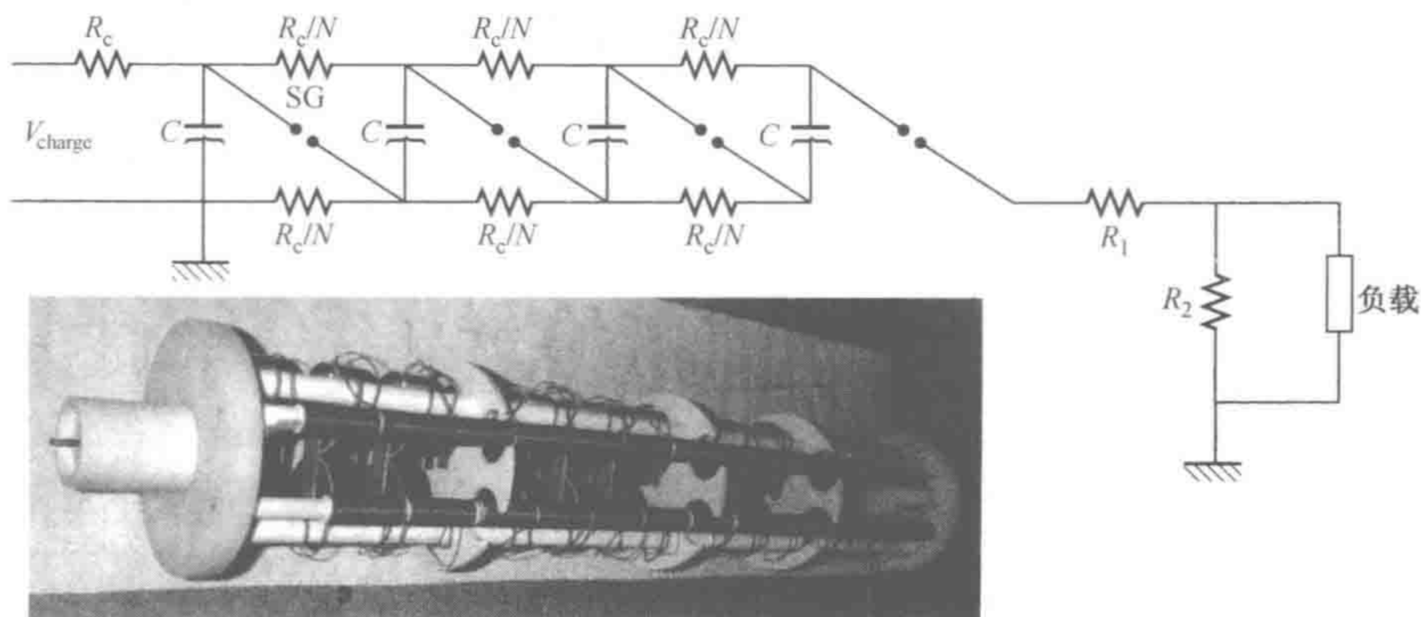
图 5 马克斯发生器原理图和实物图 (其中电容器为 13 只, 5.2\text{nF} , 40\text{kV} , 6\text{kJ/s} ; V_{\text{max}} = 350\text{kV} , 上升时间为 15\text{ns} , 脉冲宽度为 50\text{ns} , 脉冲频率为 115\text{Hz} )
