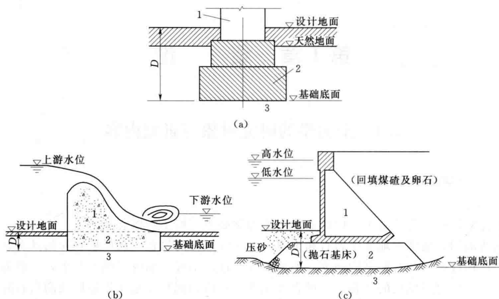
图 1-1 地基与基础示意图
