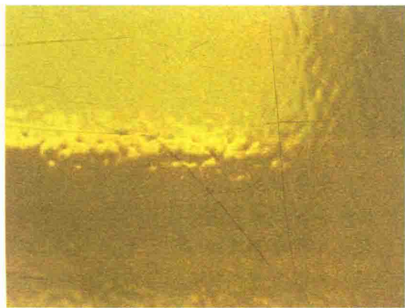
图 1-6 橘皮现象
