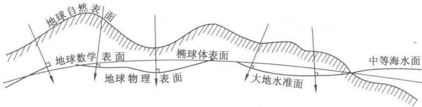
图 1-1 地球体的表面形态
