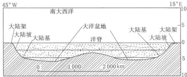
图 1-3 南大西洋海底地形示意图
