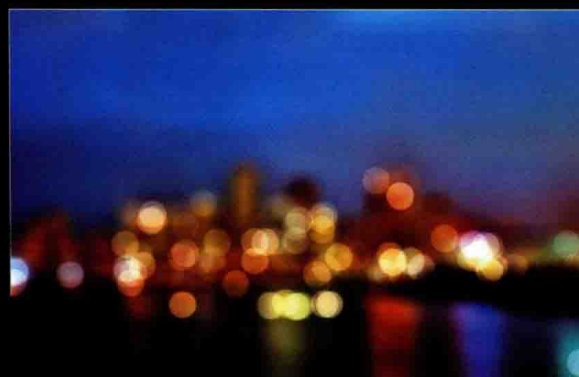
12.7.2 场景模糊
