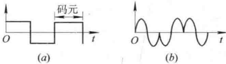
图 1-3 数字信号波形 (a) 二进制波形；(b) 2PSK 波形
