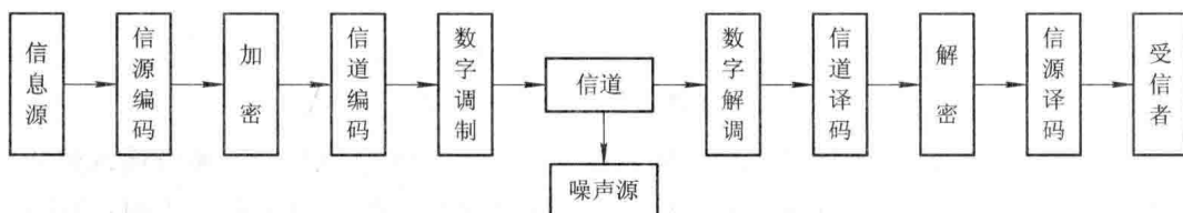
图 1-5 数字通信系统模型
