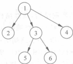
图 1.3 树形结构
