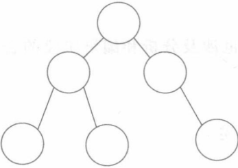
图 1.1 结构图
