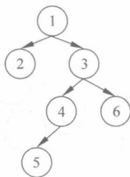
图 1.5 树形结构
