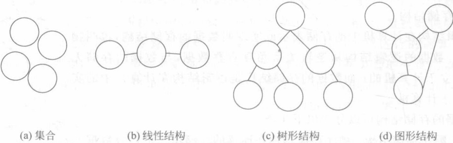
图 1.2 逻辑结构图
