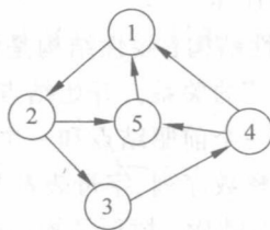
图 1.4 图形结构
