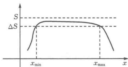
图 1-1 测量系统的动态范围定义一
