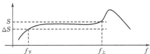
图 1-3 传感器与测量系统的频率特性
