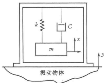
图 1-4 惯性式传感器结构原理图
