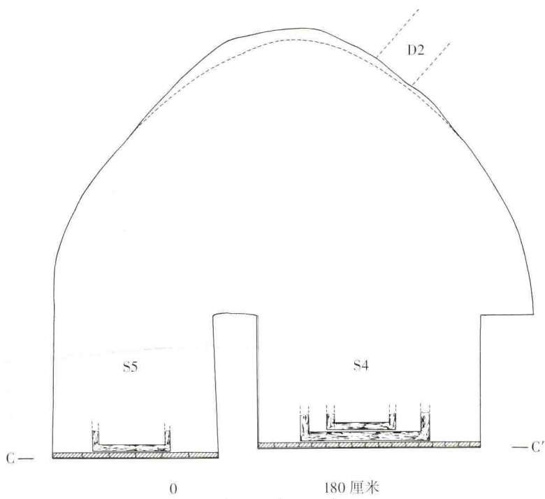
图 5-40 M2-S4、S5 横剖面图
