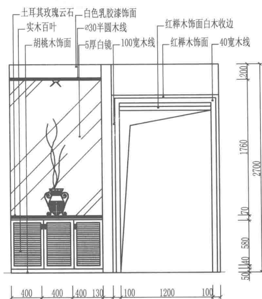
玄关柜方案5
