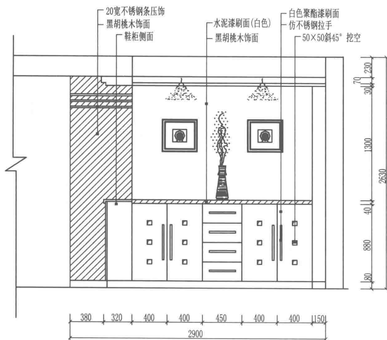
玄关柜方案24
