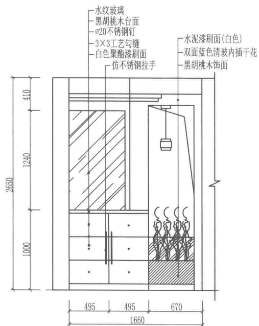
玄关柜方案19
