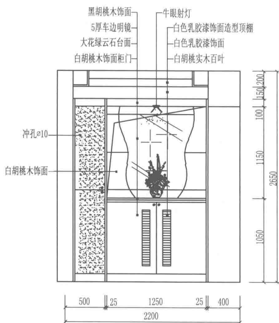
玄关柜方案17
