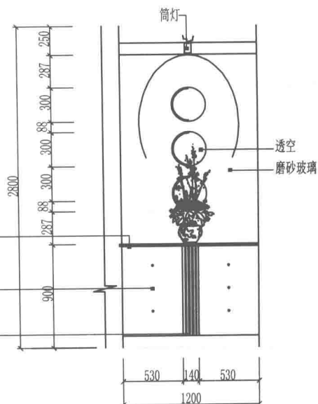
玄关柜方案29
