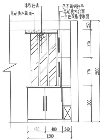
玄关柜方案6
