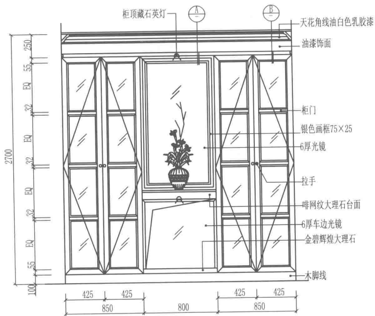
鞋柜立面图
