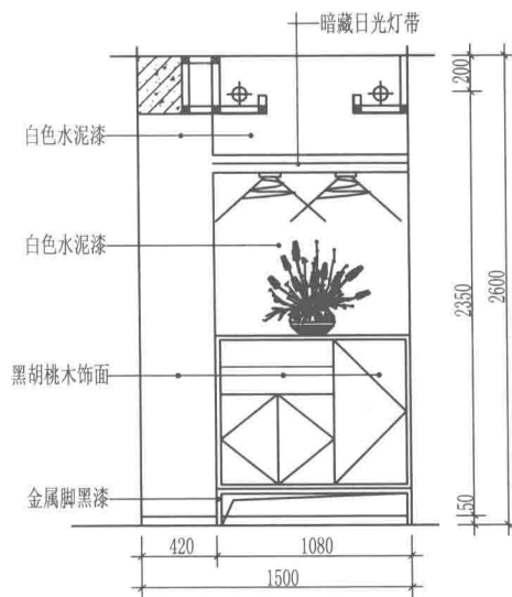
玄关柜方案14
