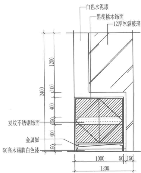
玄关柜方案16
