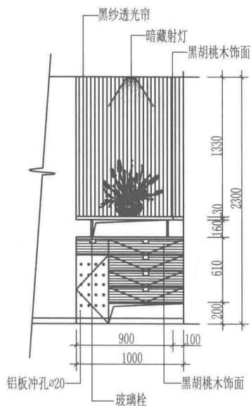
玄关柜方案2
