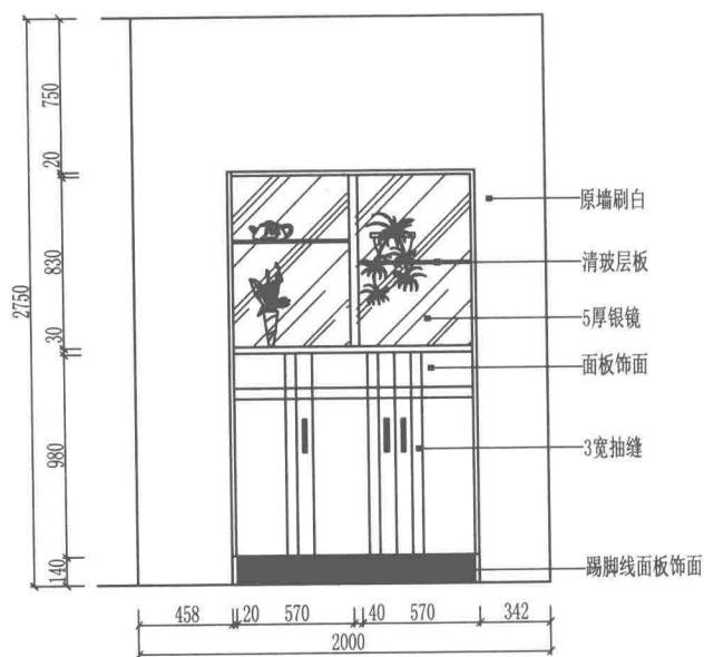
鞋柜立面图
