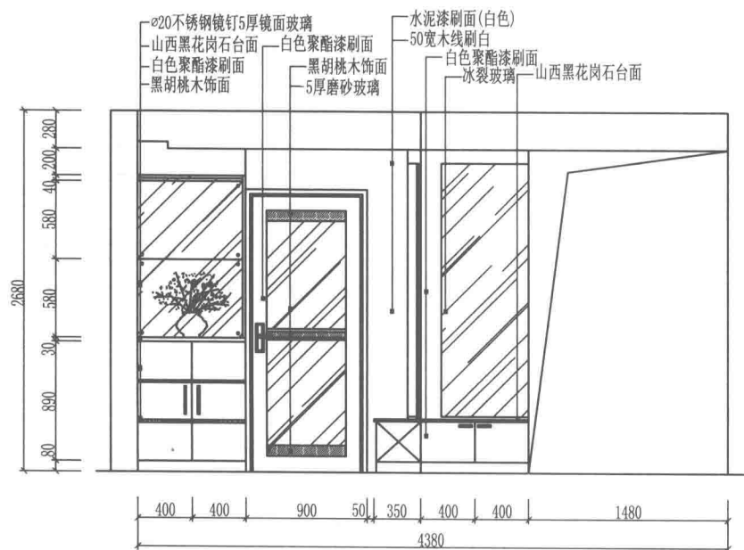
玄关柜方案25
