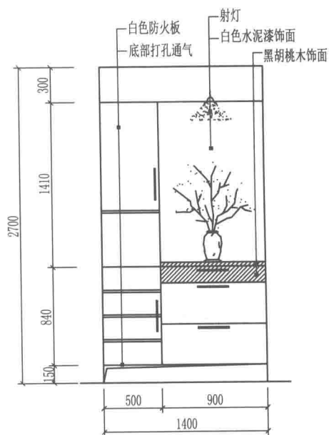
玄关柜方案27
