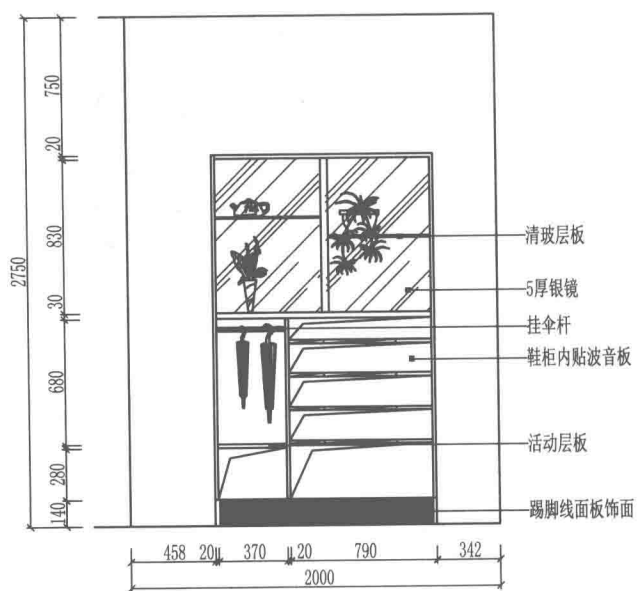
内部结构图
