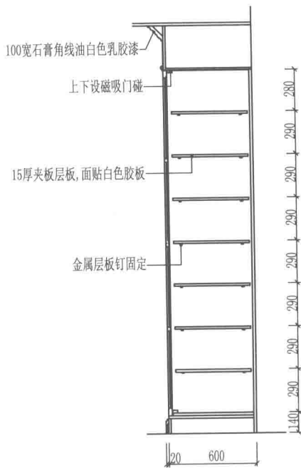
剖面图B
