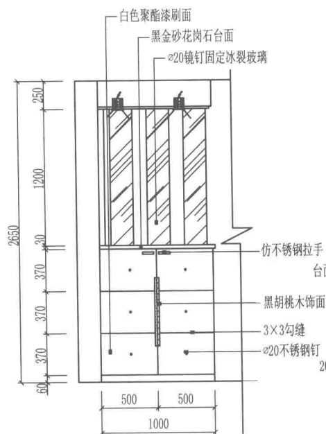
玄关柜方案28
