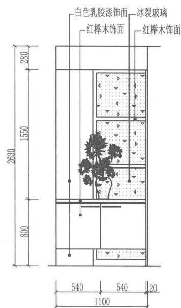
玄关柜方案18
