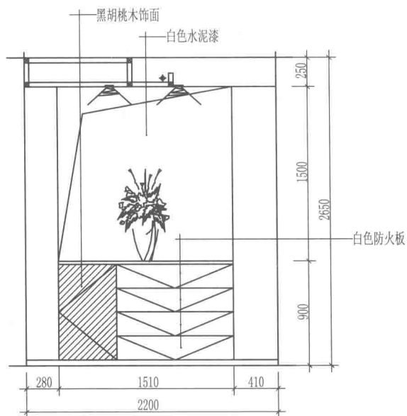
玄关柜方案15
