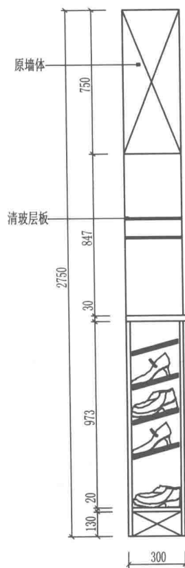
侧剖面图
