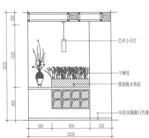
玄关柜方案13
