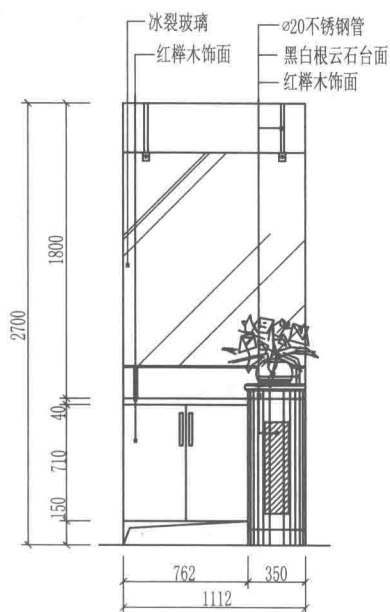
玄关柜方案4
