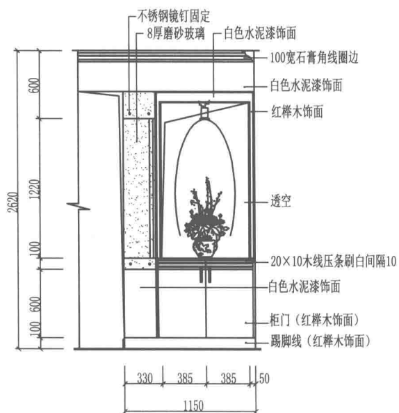
玄关柜方案11
