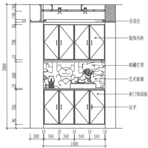
鞋柜立面图
