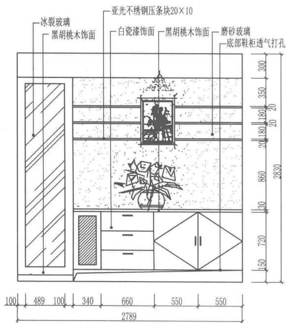
玄关柜方案3
