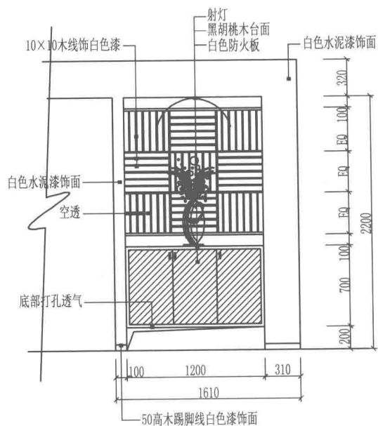
玄关柜方案26
