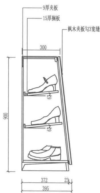
侧剖面图
