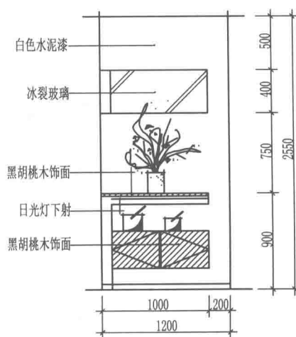
玄关柜方案8
