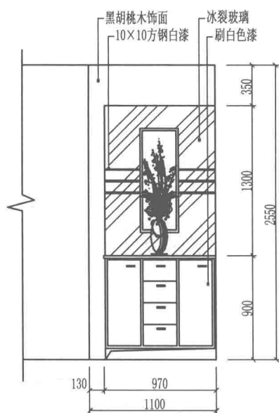
玄关柜方案9
