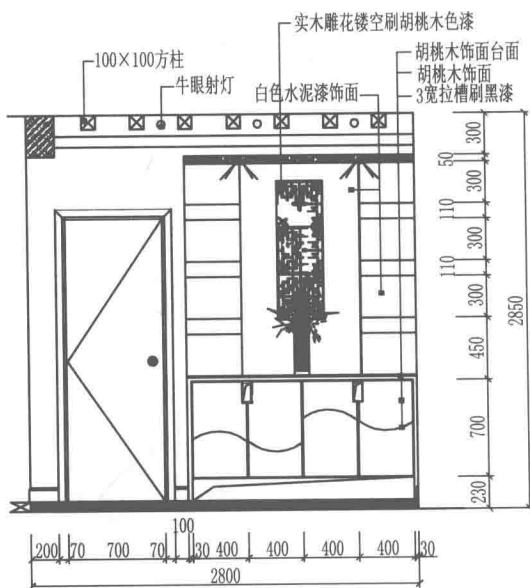
玄关柜方案22
