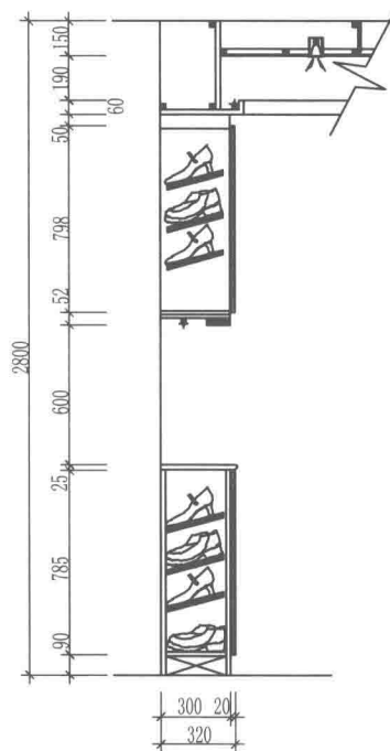
侧剖面图
