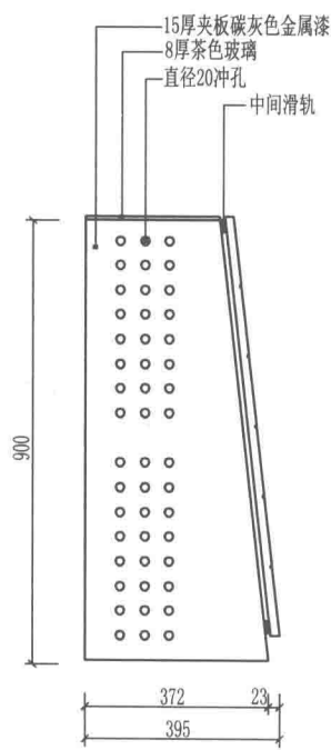
侧立面图
