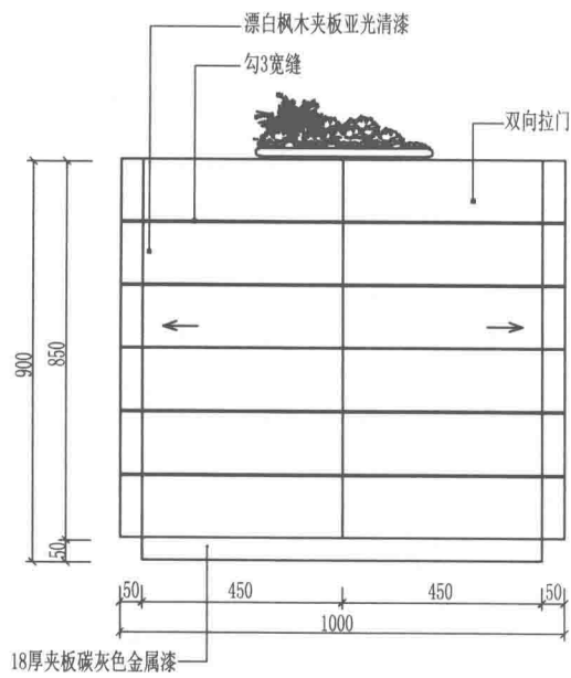
鞋柜立面图
