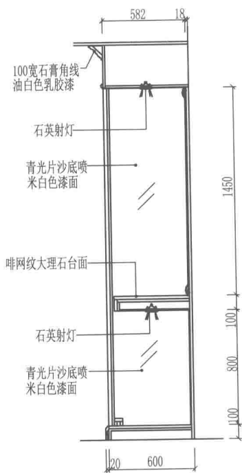
剖面图A
