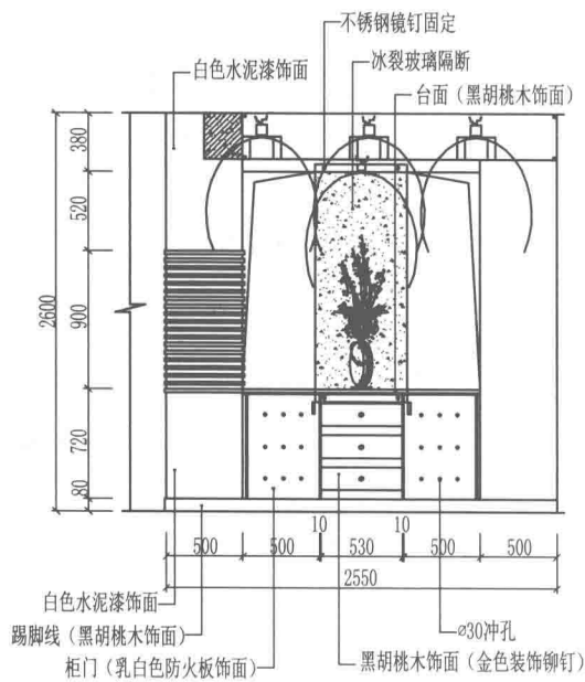
玄关柜方案1
