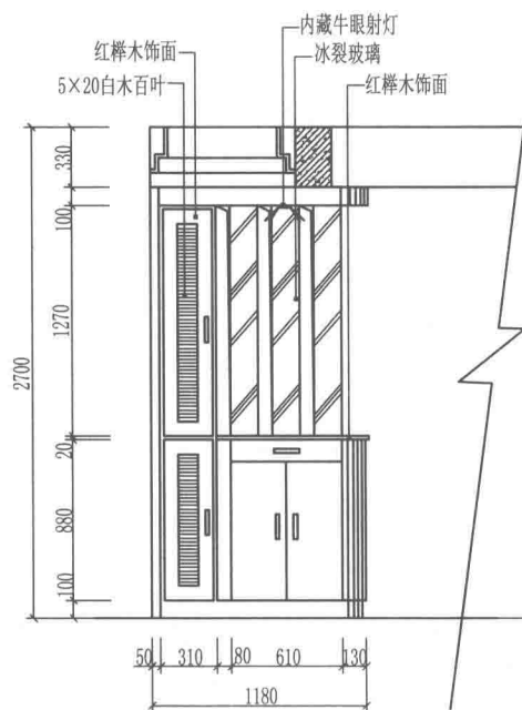
玄关柜方案10
