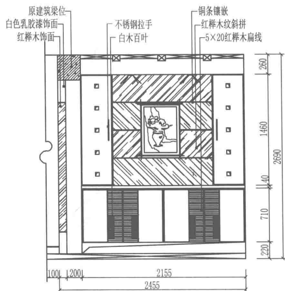
玄关柜方案7
