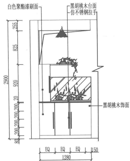
玄关柜方案23
