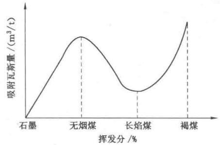
图 1-2-2 不同煤阶煤对瓦斯的吸附能力
