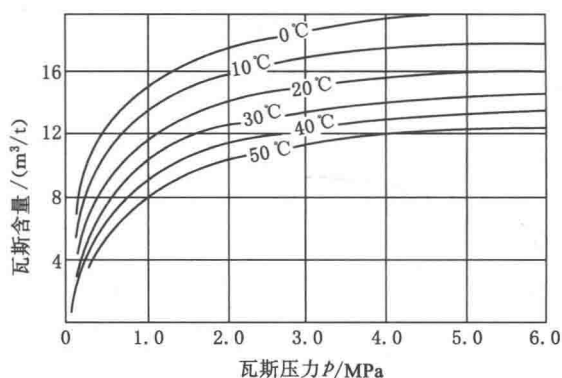
图 1-3-1 瓦斯含量与温度、瓦斯压力的关系
