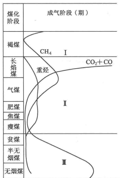
图 1-1-2 腐植煤在煤化作用阶段成气演化的一般模式 [2]
