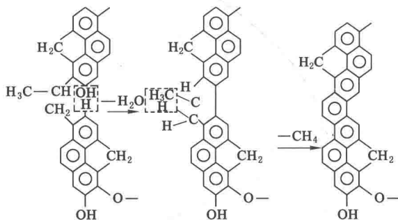
图 1-1-1 煤化作用(含碳量 83%~92%)成气反应示意图
