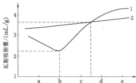
图 1-2-1 煤岩组分与瓦斯吸附量的关系
