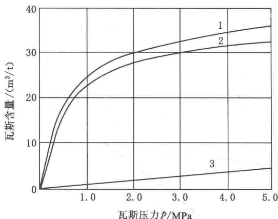
图 1-3-2 煤层瓦斯含量与瓦斯压力的关系曲线
