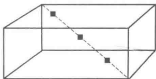
图 1-1 立体对角线布点采样法
