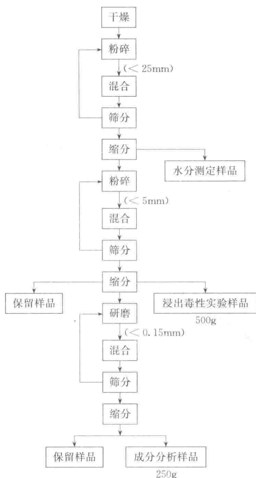
图 1-3 工业固体废物样品制备
