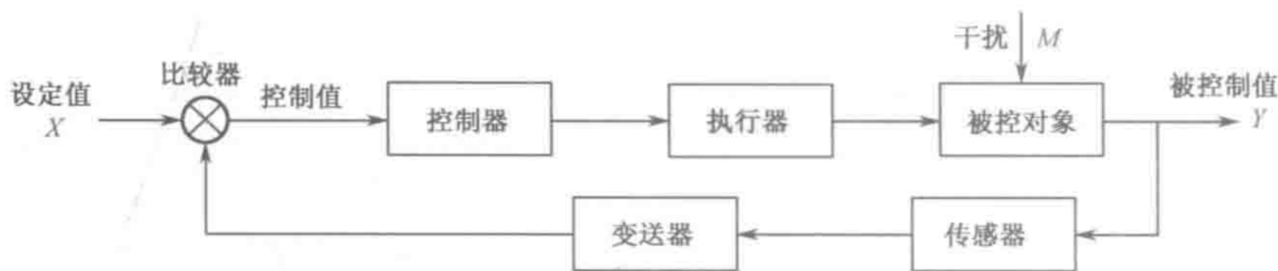
图 1-5 模拟量闭环控制系统组成框图
