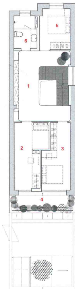
二层平面图
