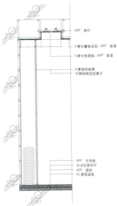
文化墙剖面图
