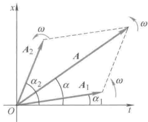
图 1-5 两个同频率简谐振动的合成
