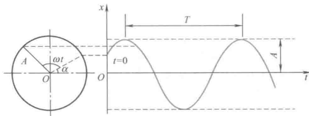
图 1-3 简谐振动的时间历程曲线
