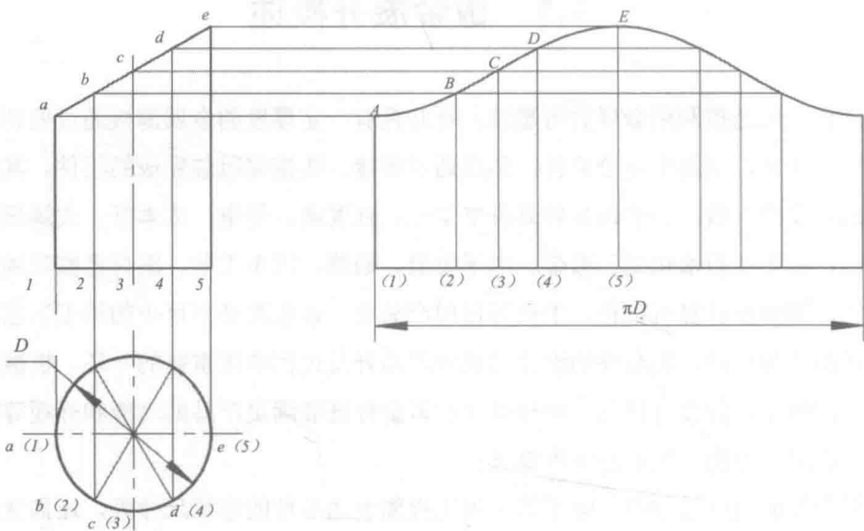
图 1.1.1 用平行线法展开斜截正圆柱面
