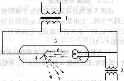
图1-1 X射线产生装置示意图
