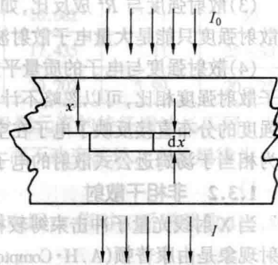
图 1-4 X 射线穿过物质时被衰减
