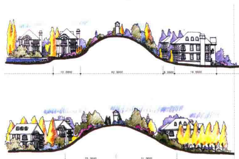
中心水景剖面图
