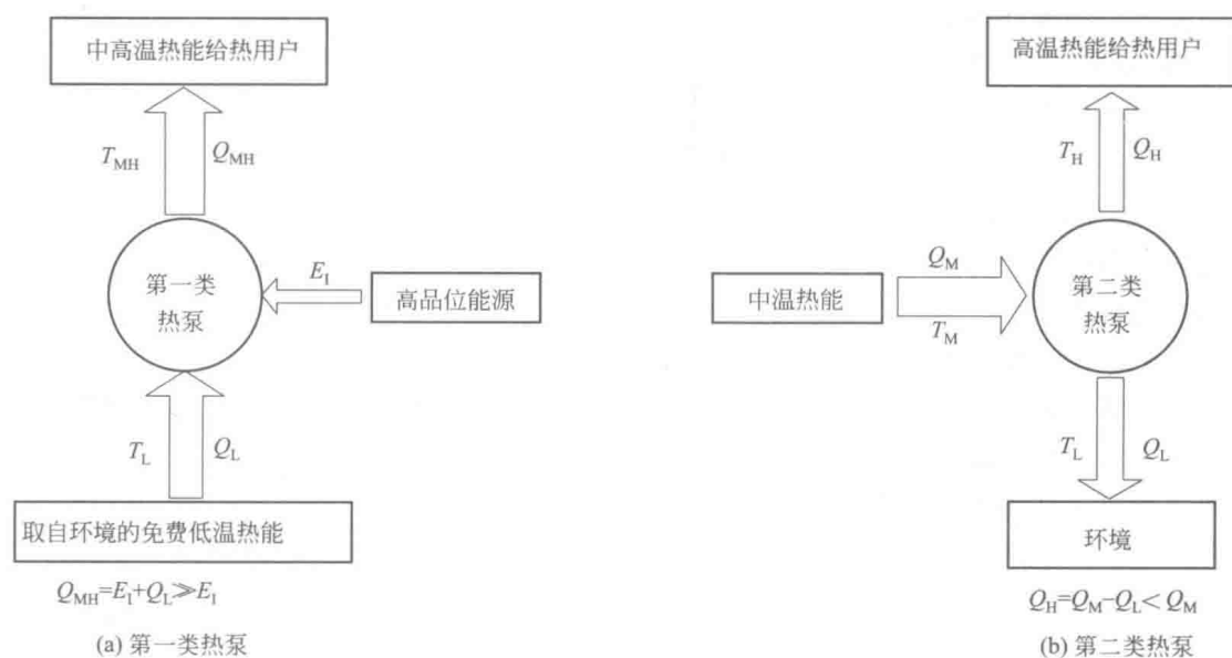
图 1-3 第一类热泵和第二类热泵示意
