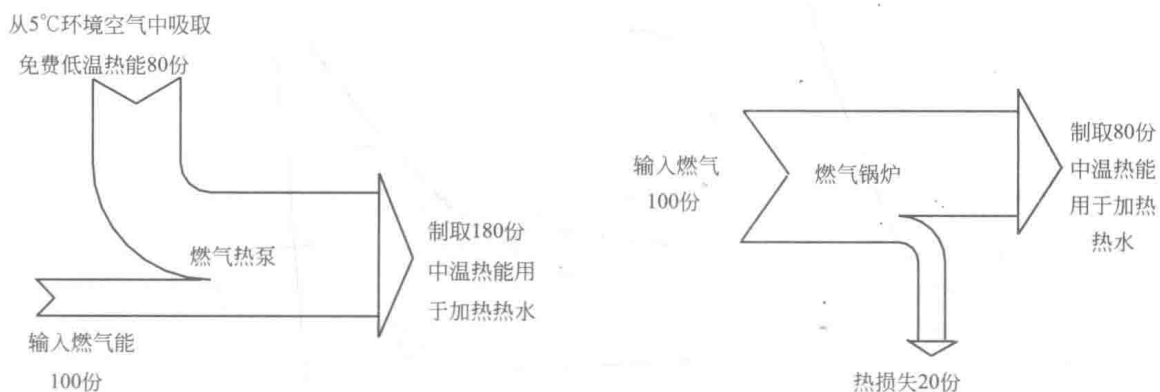
(b) 燃气热泵与燃气锅炉的能流图
