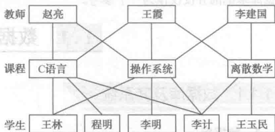
图 1.3 按网状模型组织的数据示例
