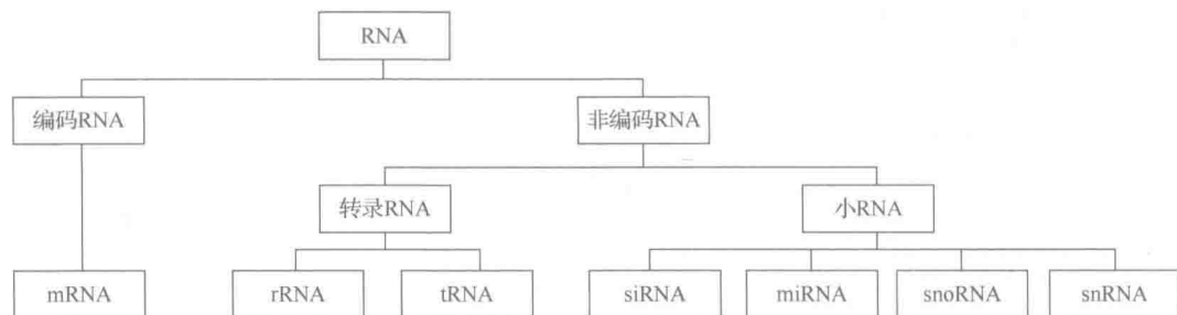
图 1-1 RNA 的分类
