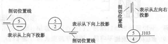
图 1-5 索引剖面详图的索引符号
