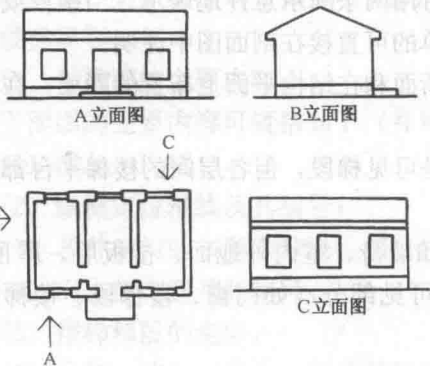
图 1-15 建筑立面图的形成
