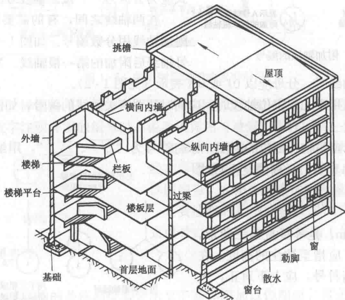
图 1-1 房屋的基本组成
