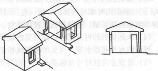
图 1-14 建筑剖面图的形成
