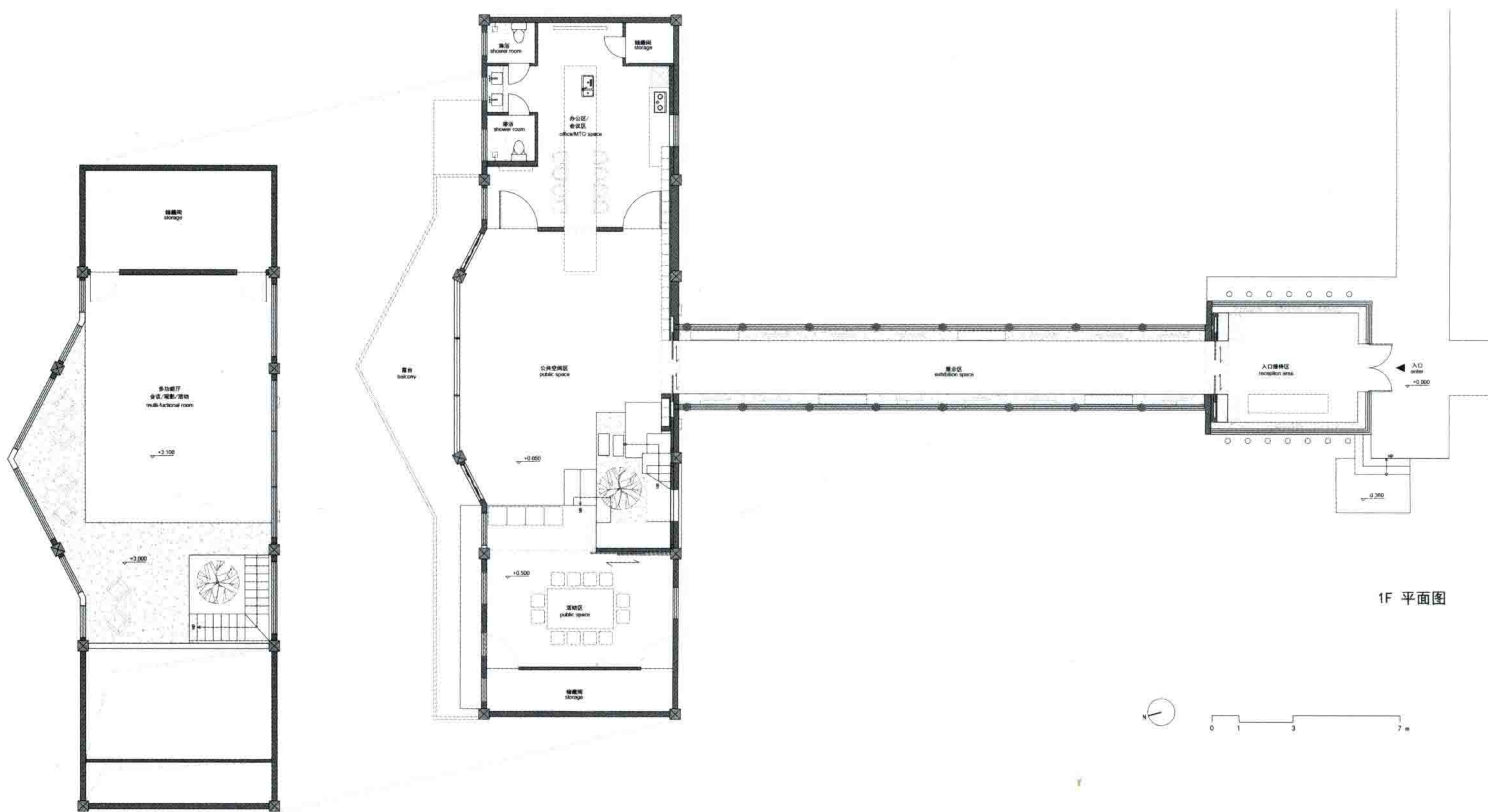
2F 平面图
