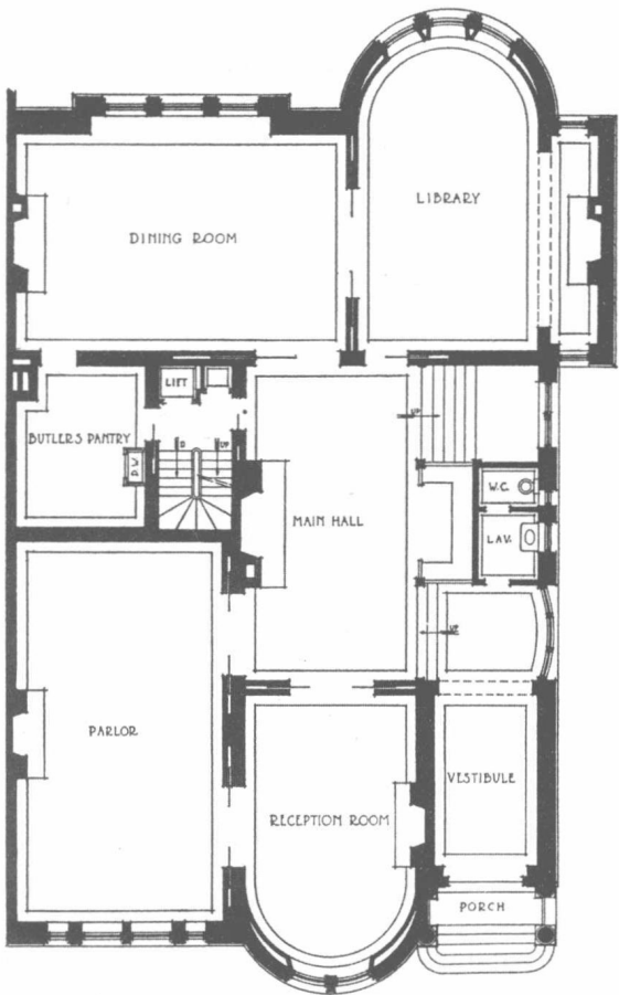
一层平面图
