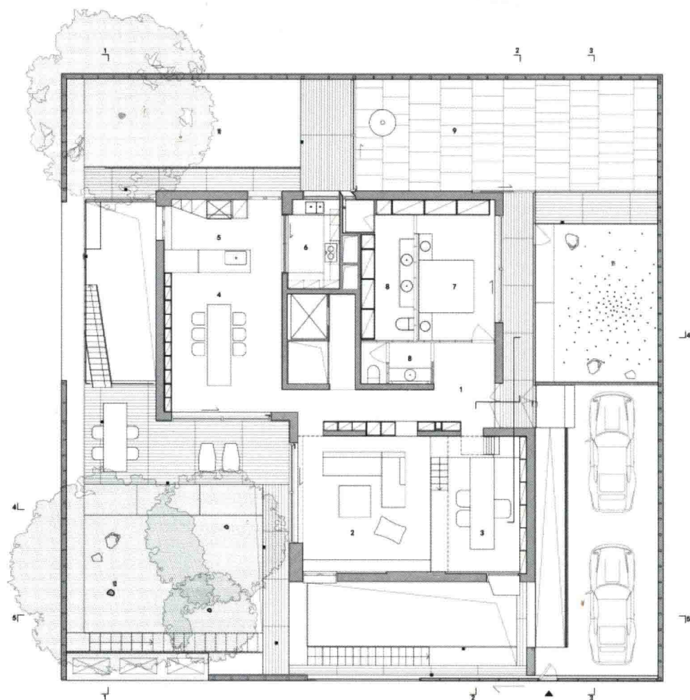
一层平面图
