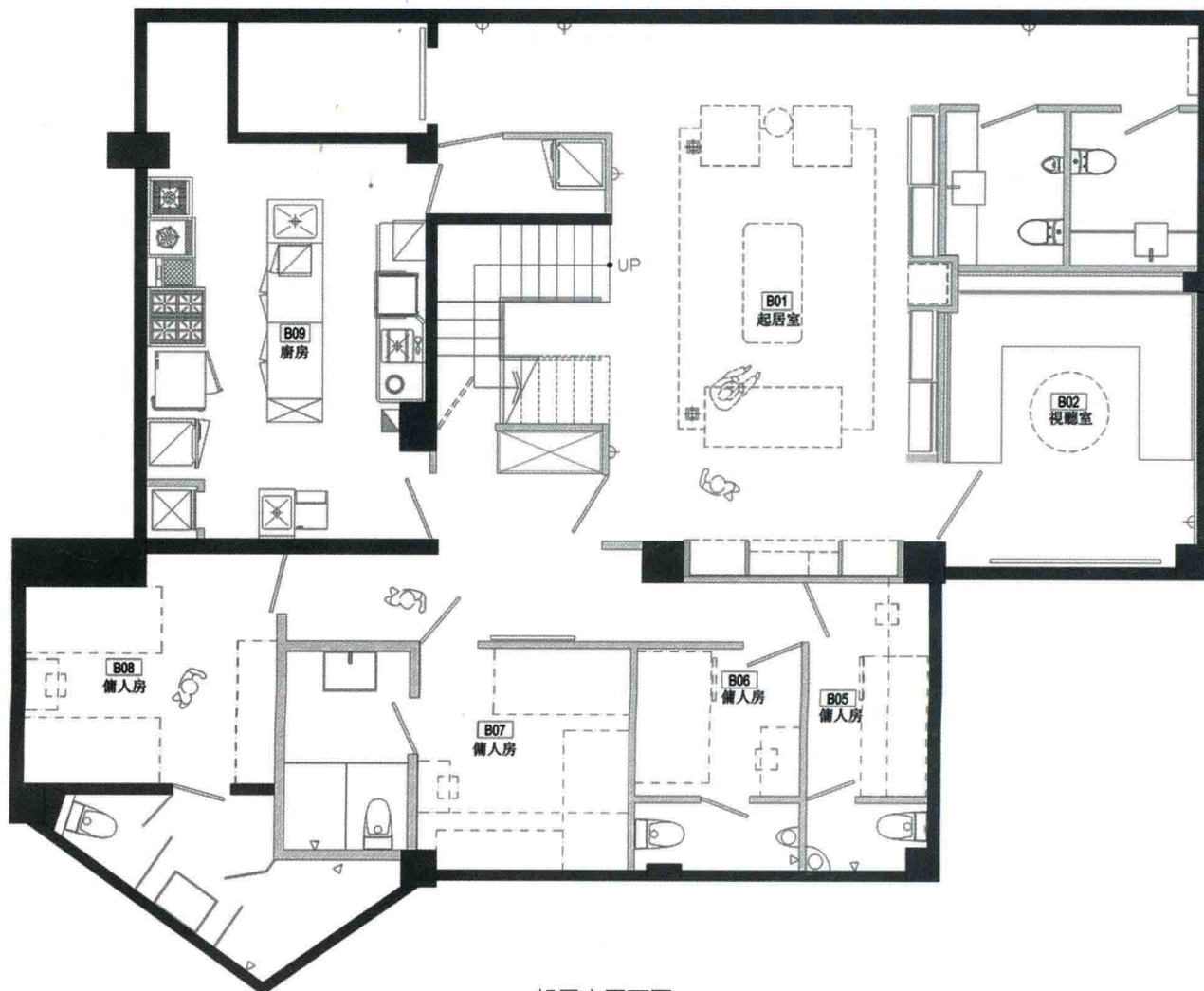
起居室平面图
