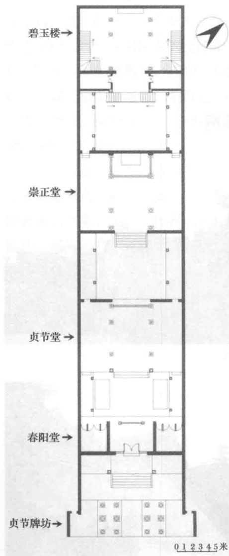
白沙祠建筑平面图
