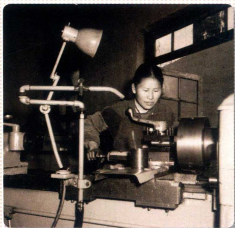
20世纪70年代茅台酒厂金工班使用的车床
