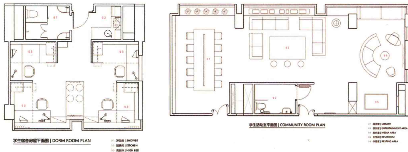
图 1-13 学生公寓宿舍和活动室平面图
