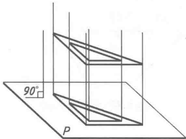
图 1-4 正投影
