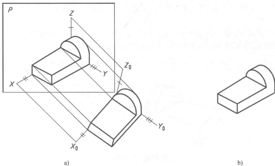
图 1-13 轴测投影
