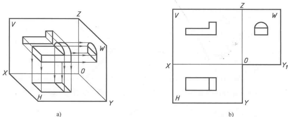
图 1-12 物体的正投影
