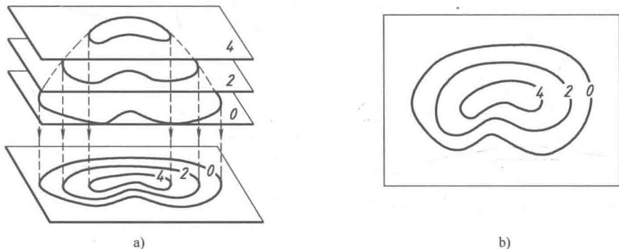
图 1-14 标高投影
