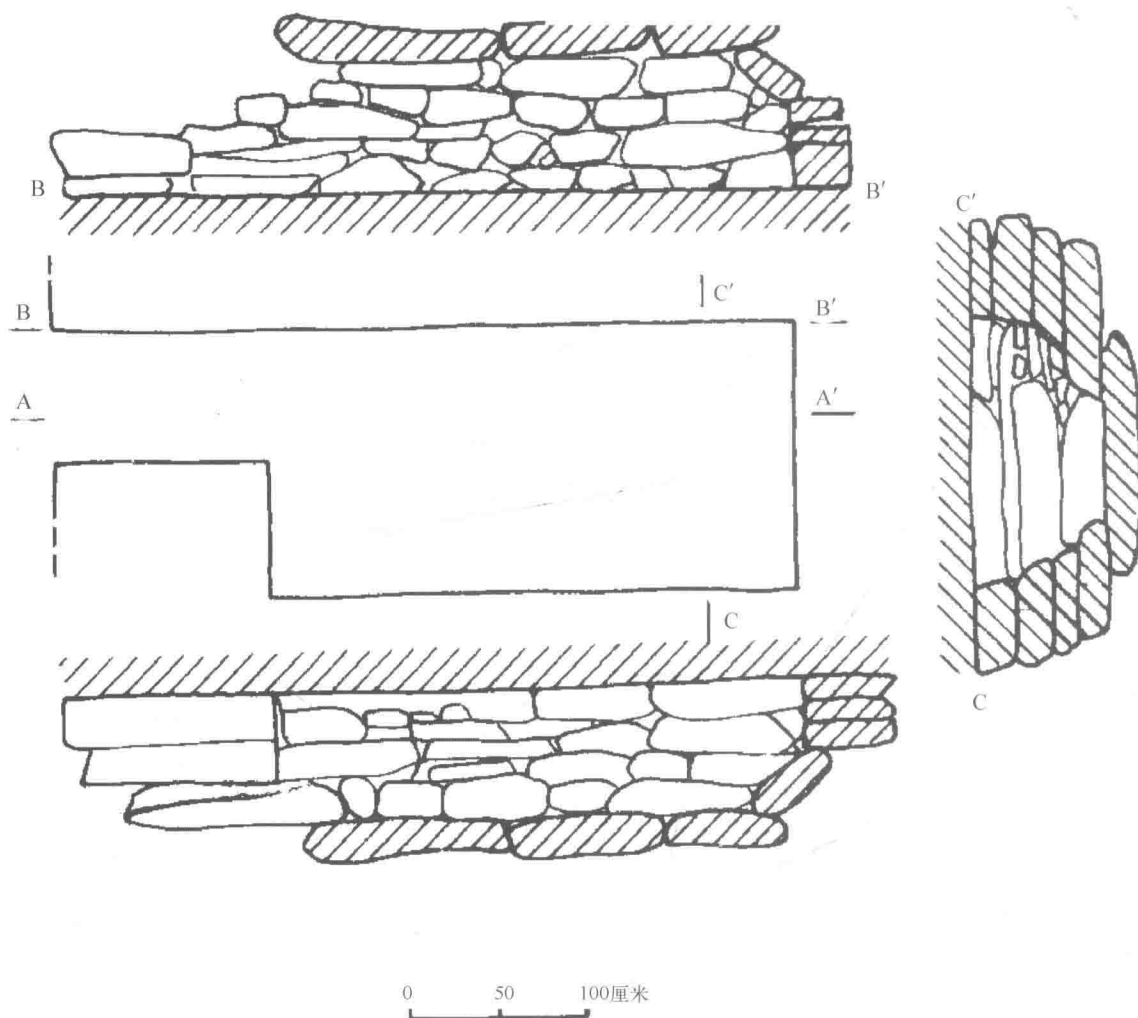
南云台山M17封土石室墓测绘图
