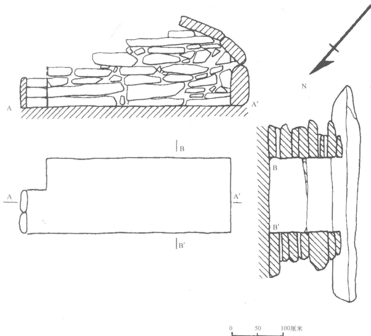
南云台山M12封土石室墓测绘图
