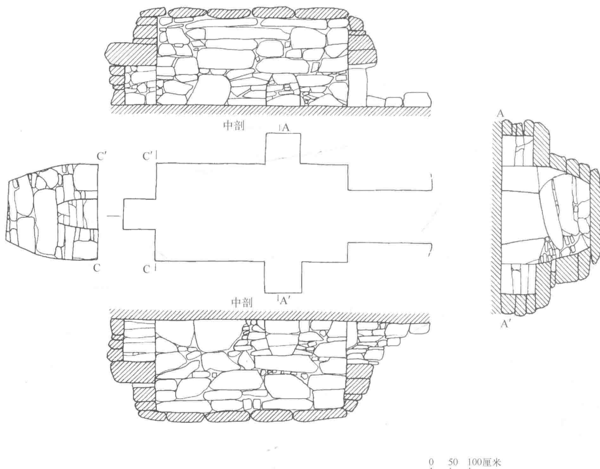
南云台山M37封土石室墓测绘图
