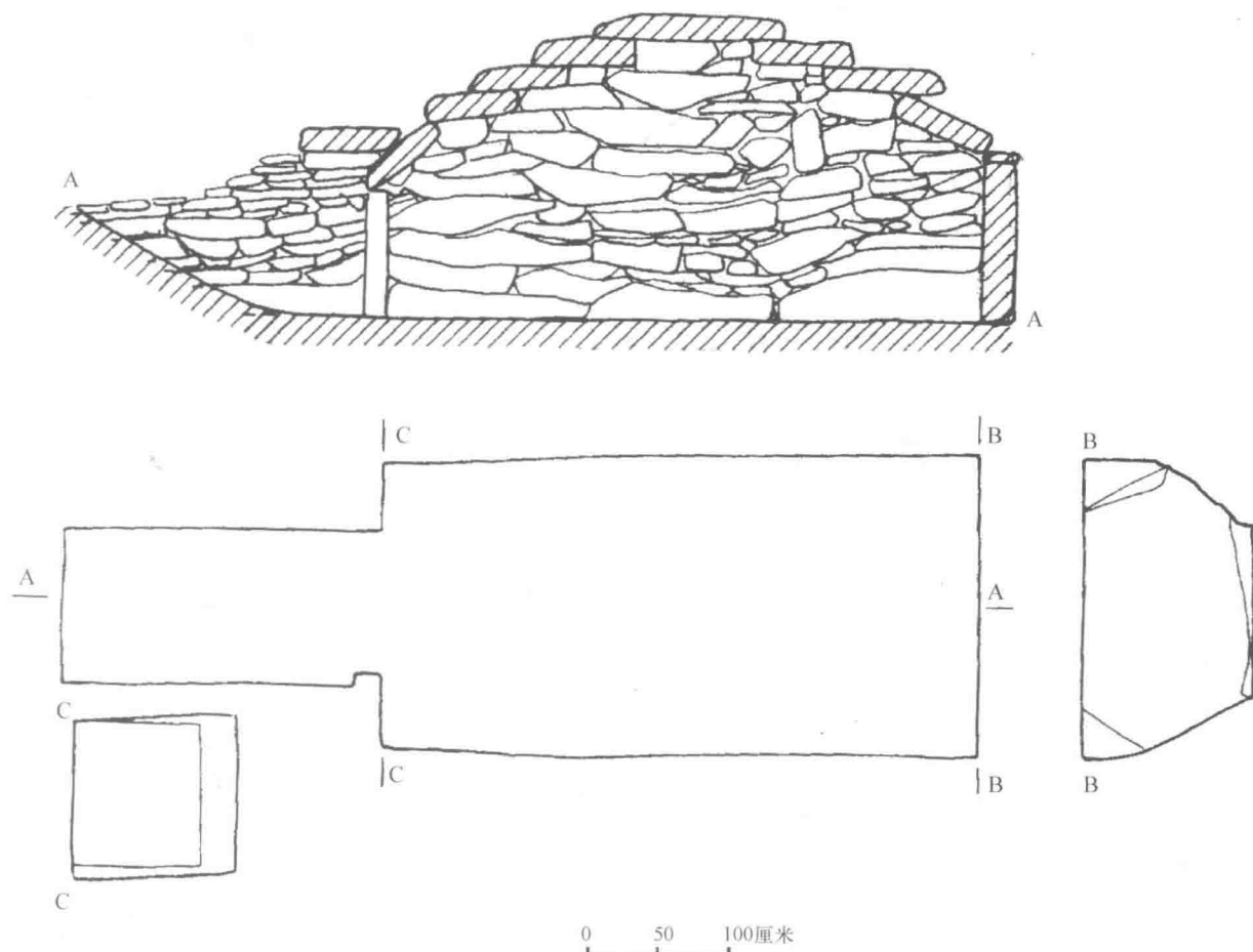
南云台山M70封土石室墓测绘图
