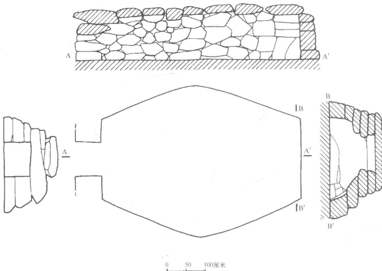
南云台山M2封土石室墓测绘图
