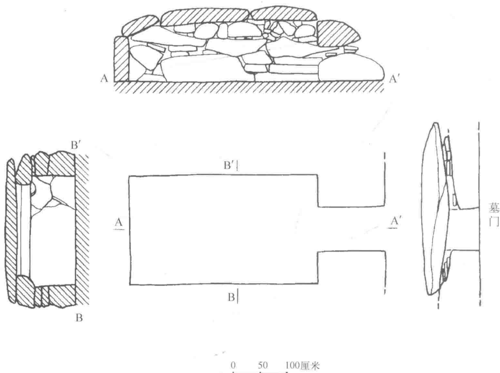
南云台山M15封土石室墓测绘图
