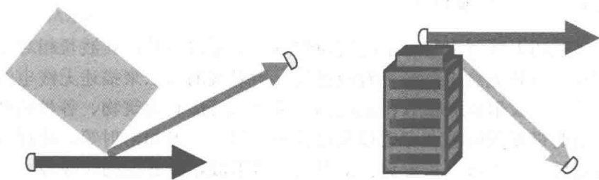
图 1-2 衍射示意图
