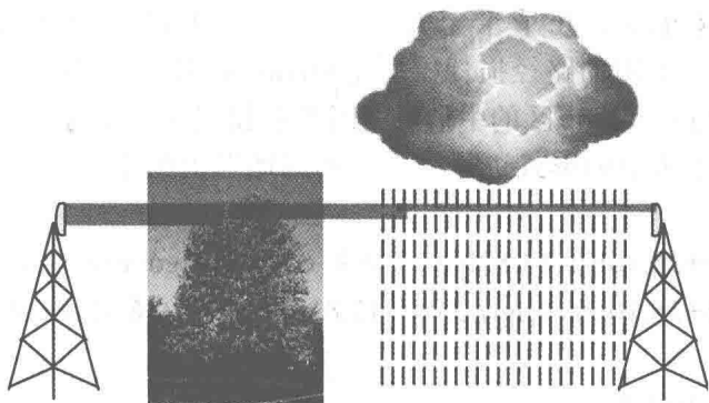
图 1-3 吸收示意图
