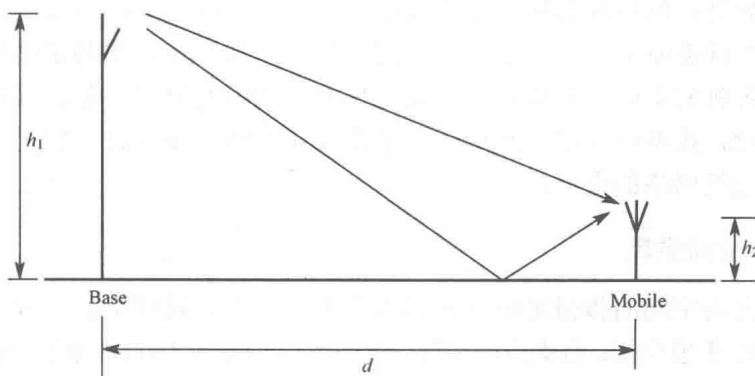
图 1-4 无线电波传播模型示意图
