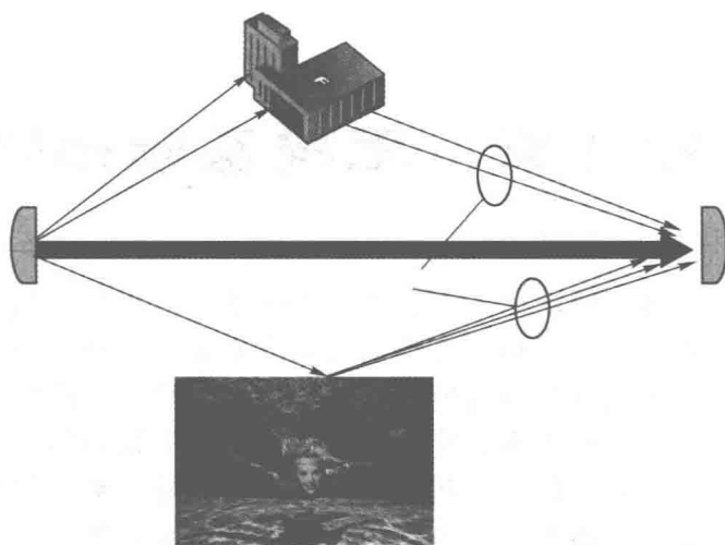
图 1-1 反射示意图
