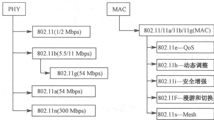
图 2-2 802.11 标准的划分
