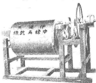
機乾再葉茶
