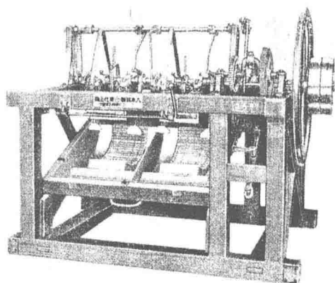
機揉精葉茶
