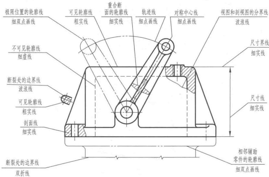
图 1-11 图线应用举例
