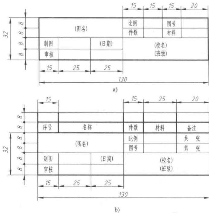
图 1-4 制图作业用标题栏
