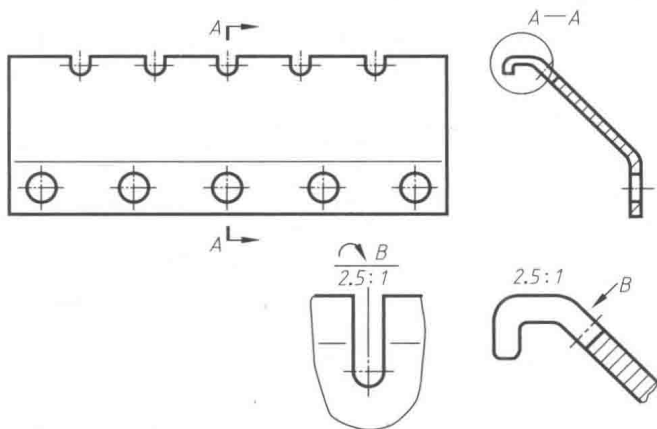
图 1-6 不同比例的视图应加标注
