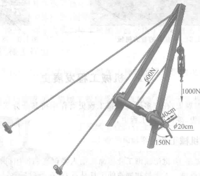
图 1.1 维托洛维斯定义的机械(起重机)
