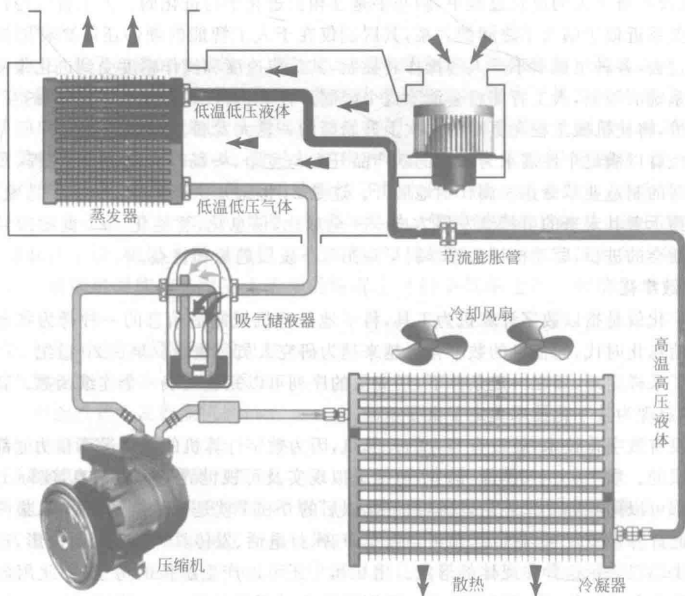
图 1.11 汽车空调原理图
