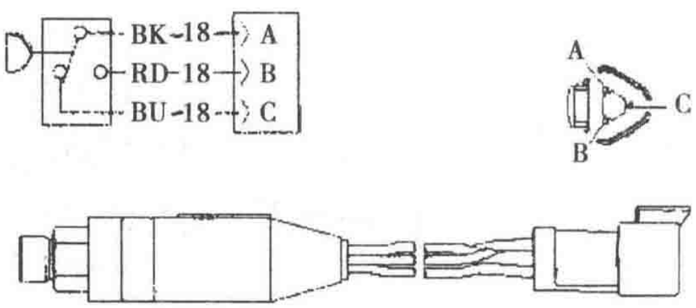
图 1-1-9 发动机机油压力开关
