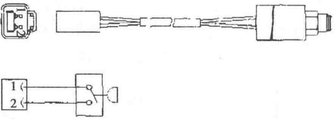
图 1-1-10 动臂提升压力开关
