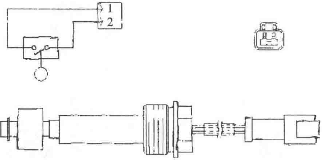
图 1-1-11 发动机机油油位开关
