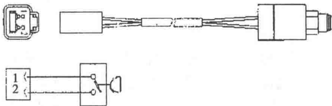
图 1-1-6 输送压力开关和机具/转盘压力开关
