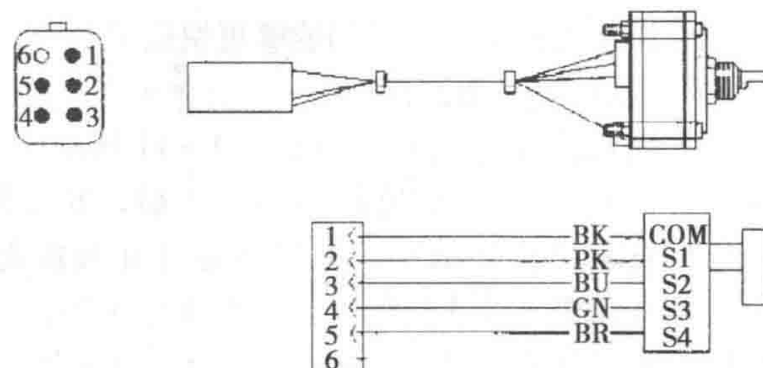
图 1-1-5 发动机转速旋钮开关
