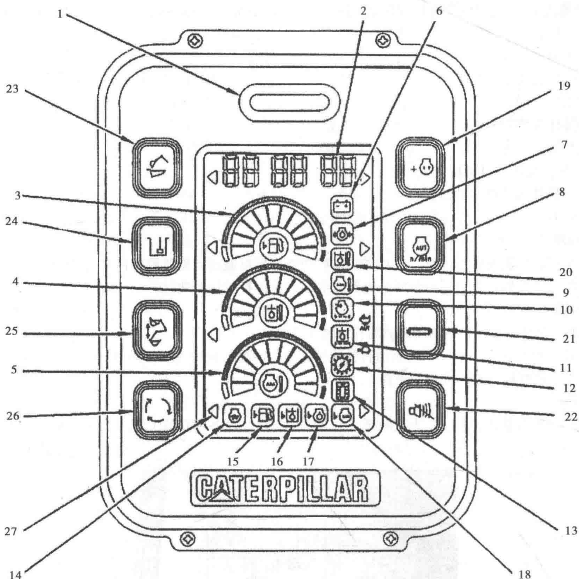
1 - 作用指示灯 2 - 字符显示屏 3 - 燃油表 4 - 液压油温度表 5 - 发动机冷却液温度表 6 - 充电报警指示器 7 - 发动机机油压力报警灯 8 - 液压油温度报警灯 9 - 发动机冷却液温度报警灯 10 - 空气滤清器堵塞指示灯 11 - 液压油回油过滤器堵塞指示灯 12 - 控制器报警指示灯 13 - 监控器报警指示灯 14 - 空气加热器指示灯 15 - 燃油油位报警指示灯 16 - 液压油油位报警指示灯 17 - 发动机机油油位报警指示灯 18 - 发动机冷却液液面报警指示灯 19 - 动力模式开关 20 - AEC (自动转速控制) 开关 21 - 行驶速度控制开关 22 - 行车报警解除开关 23 - 大臂优先模式开关 24 - 回转优先模式开关 25 - 微调 (整平) 控制模式开关 26 - 用户自定义模式开关 27 - 仪表指示符号
