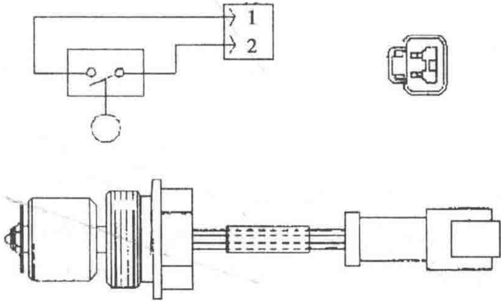
图 1-1-8 液压油油位开关
