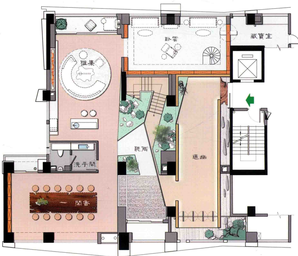
一层平面图
