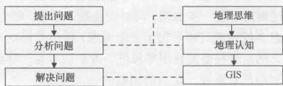
图 1-4 地理认知、地理思维和 GIS 的关系
