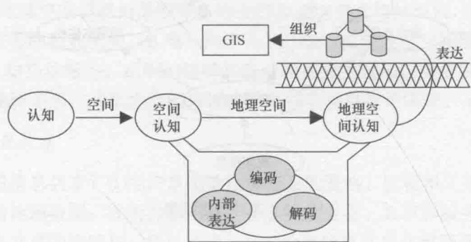
图 1-3 GIS 与空间认知关系
