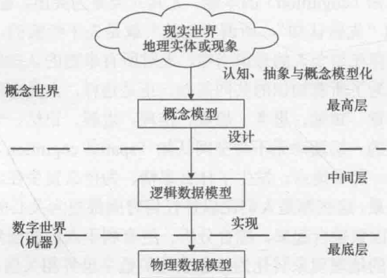
图 1-2 认知模型
