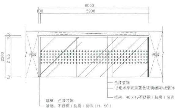
立面图J
