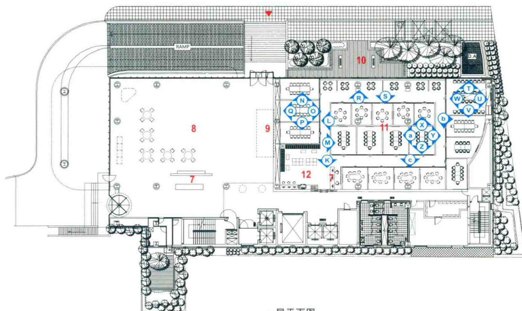
一层平面图
