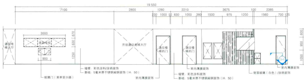
立面图A
