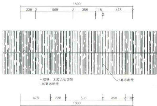
细节图A
