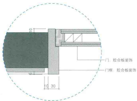
剖面图C
