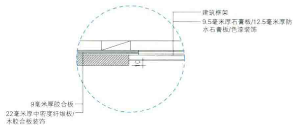
剖面图B
