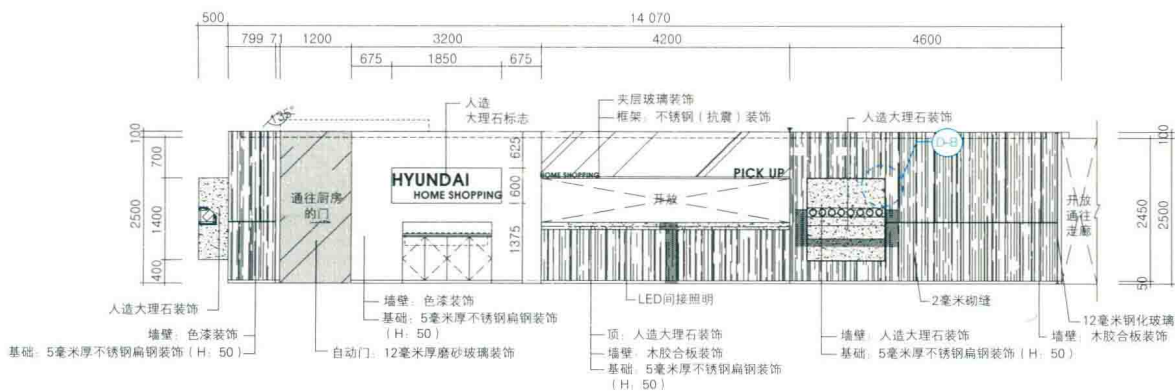
立面图C
