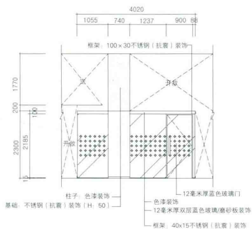
立面图I
