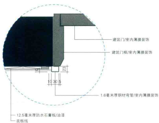
剖面图A
