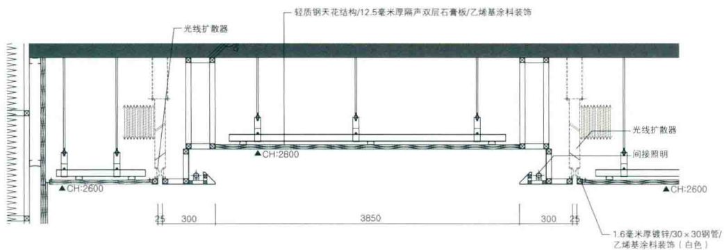
细节图C
