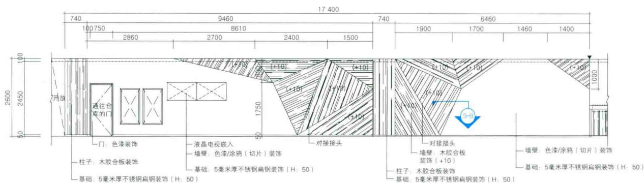
立面图D
