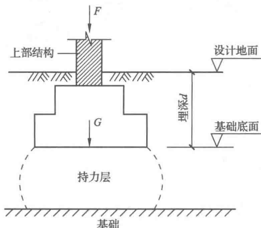
图 0-1 地基及基础示意图
