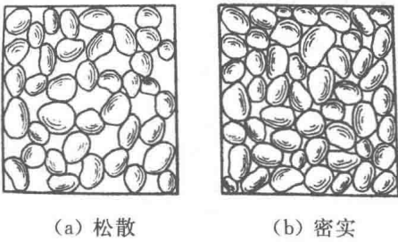
图 1-1 土的单粒结构
