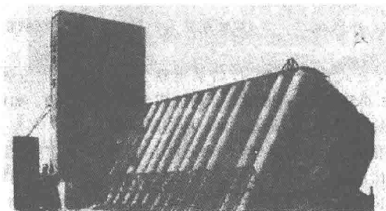
图 0-2 加拿大特朗斯康谷仓的地基事故
