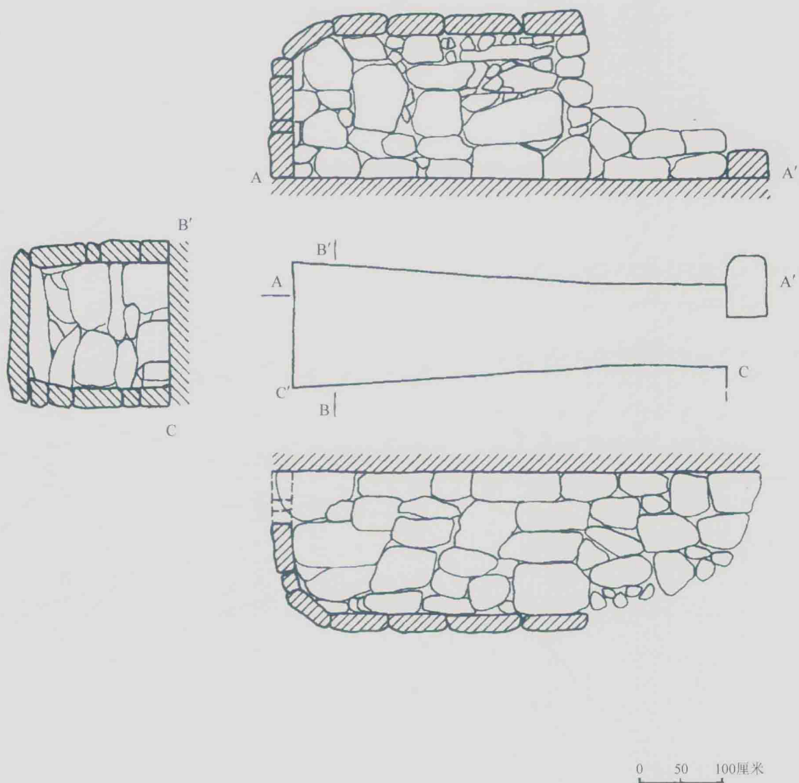
0001 • JPSM001 封土石室墓测绘图
