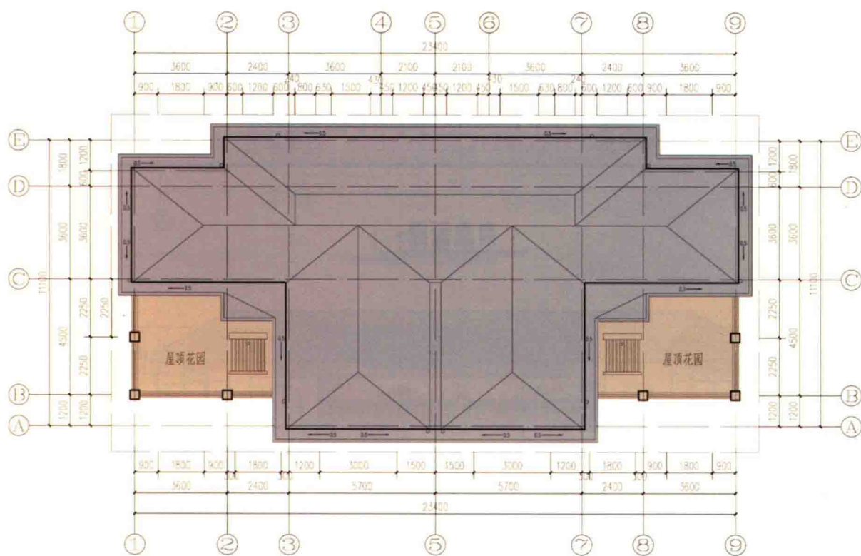
屋面排水布置图
