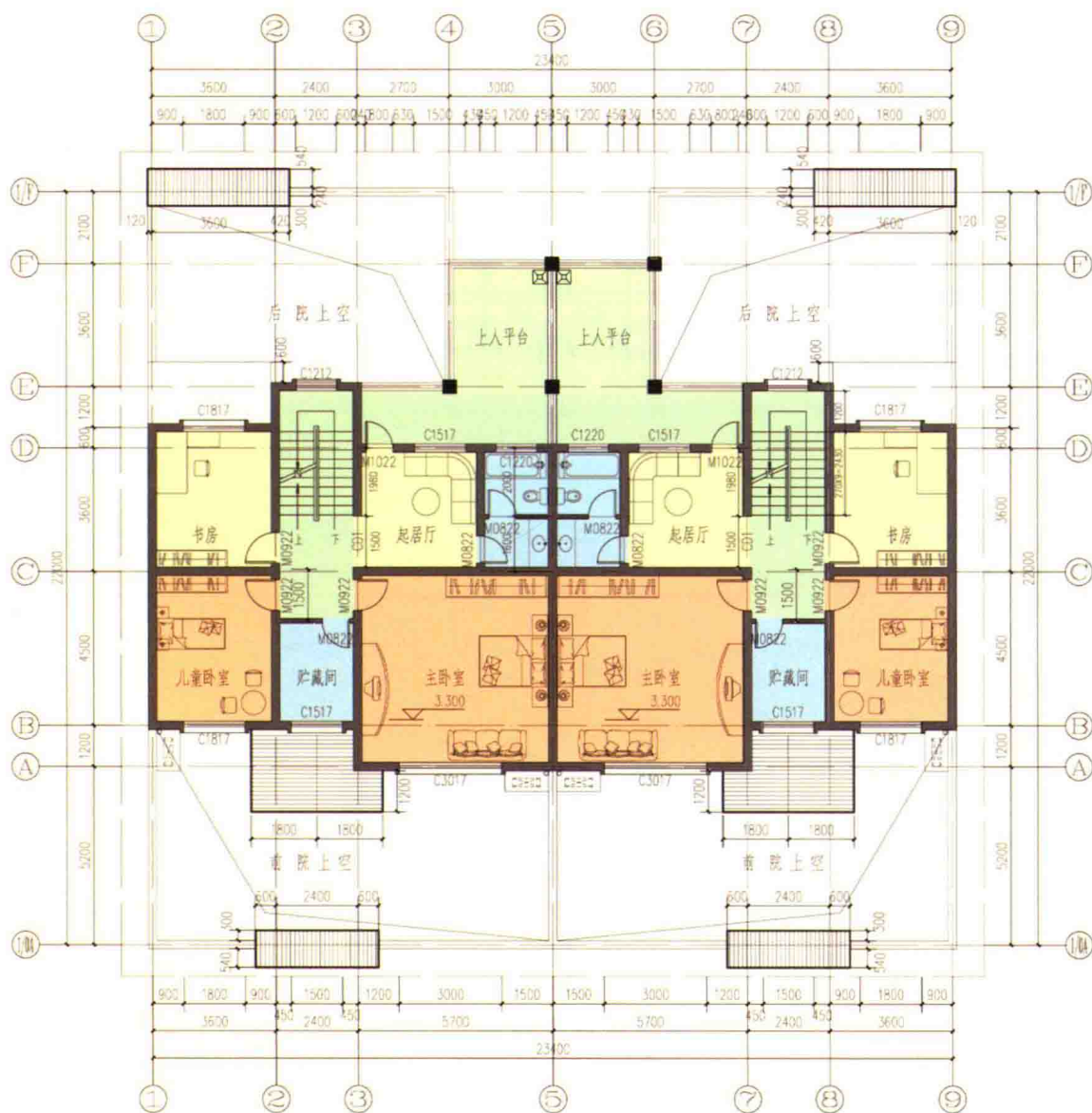
二层平面图
