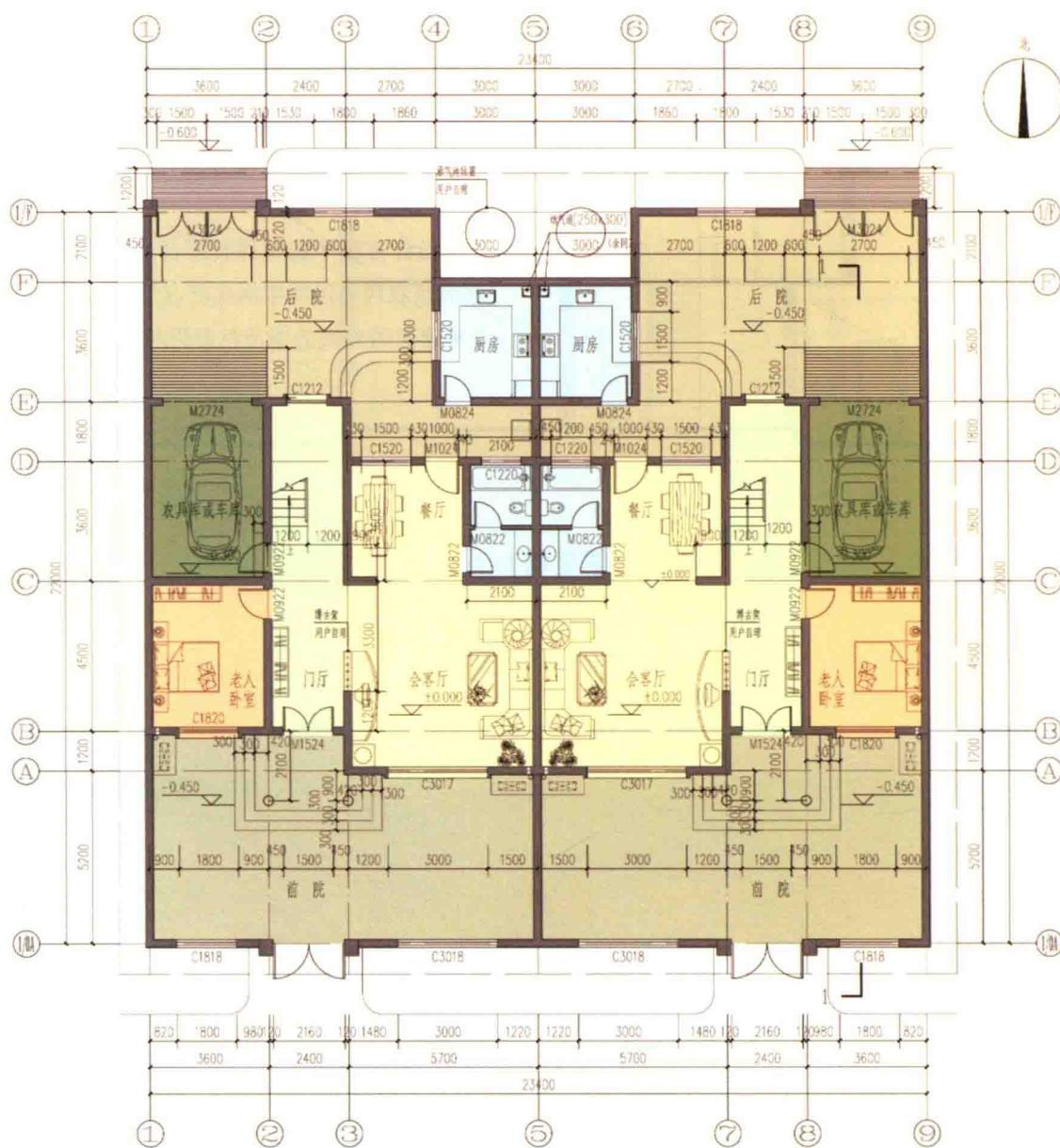
一层平面图
