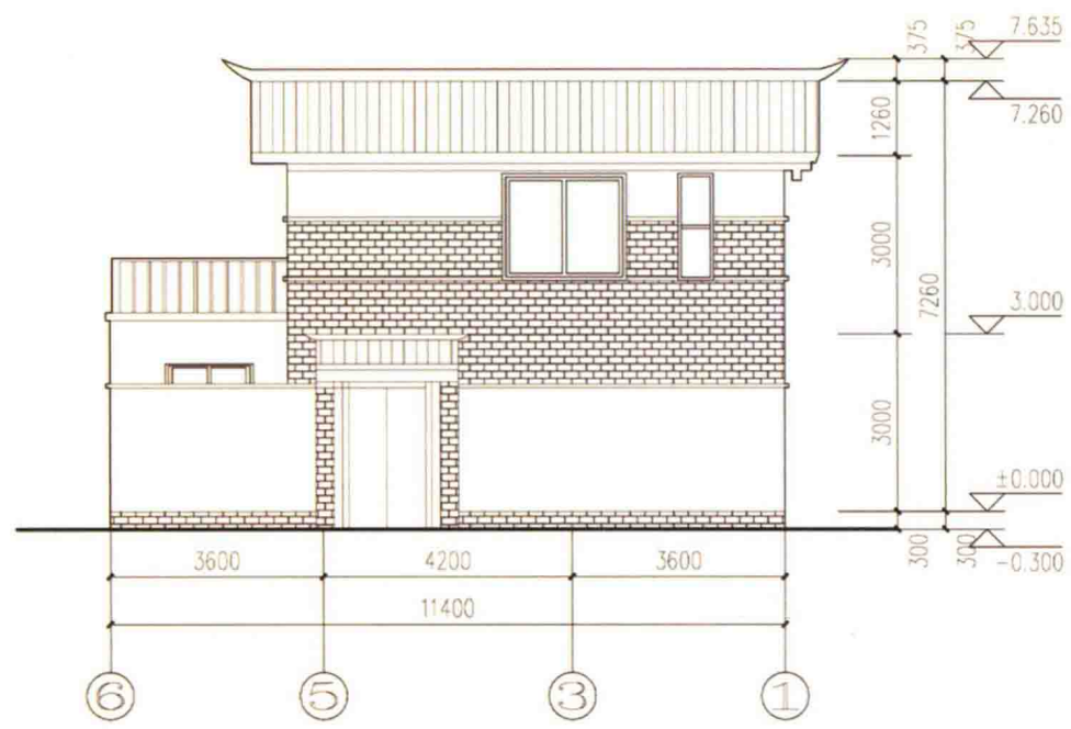
⑥-①立面图
