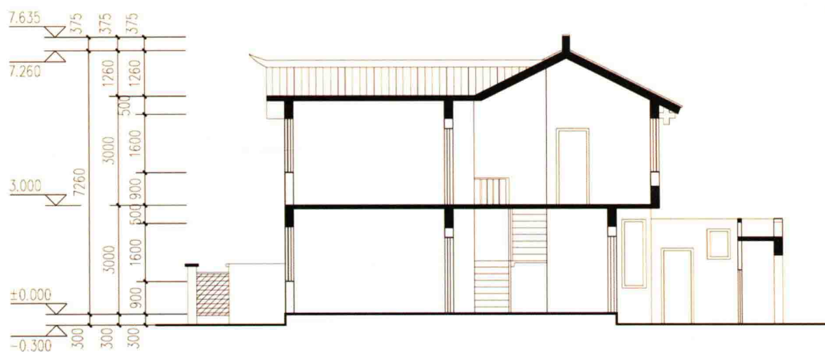
1-1剖面图
