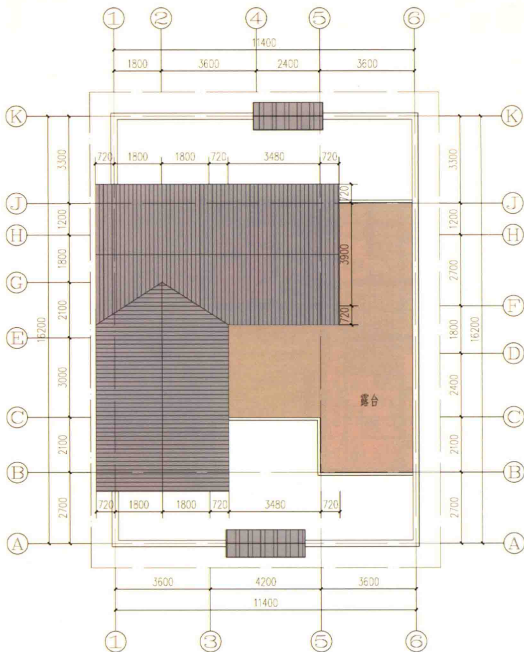
屋顶平面图
