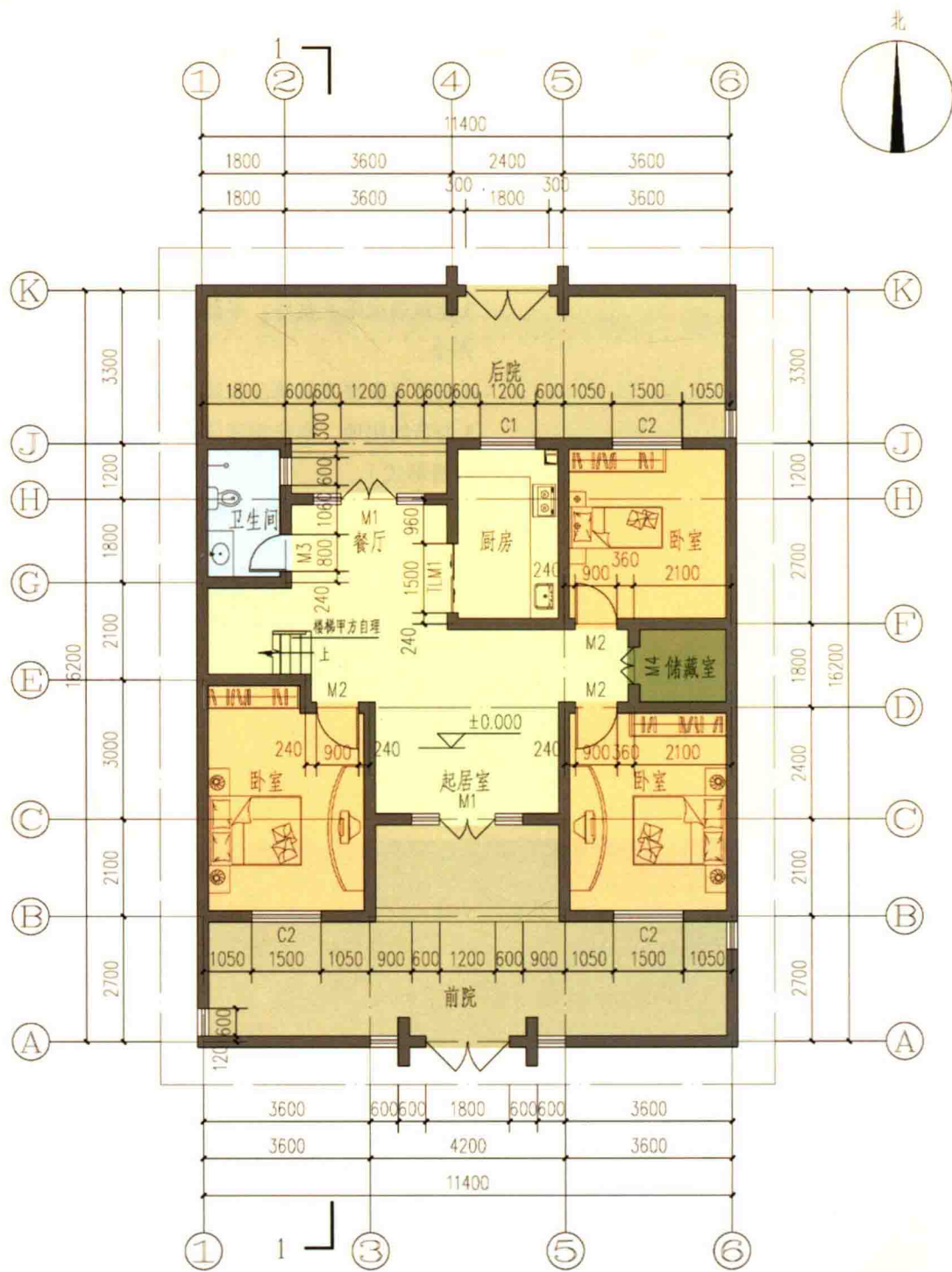
一层平面图
