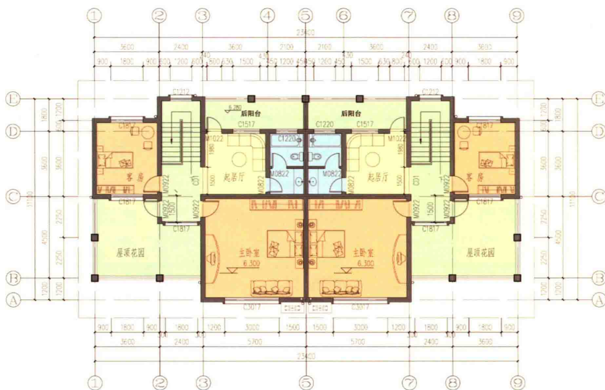
三层平面图
