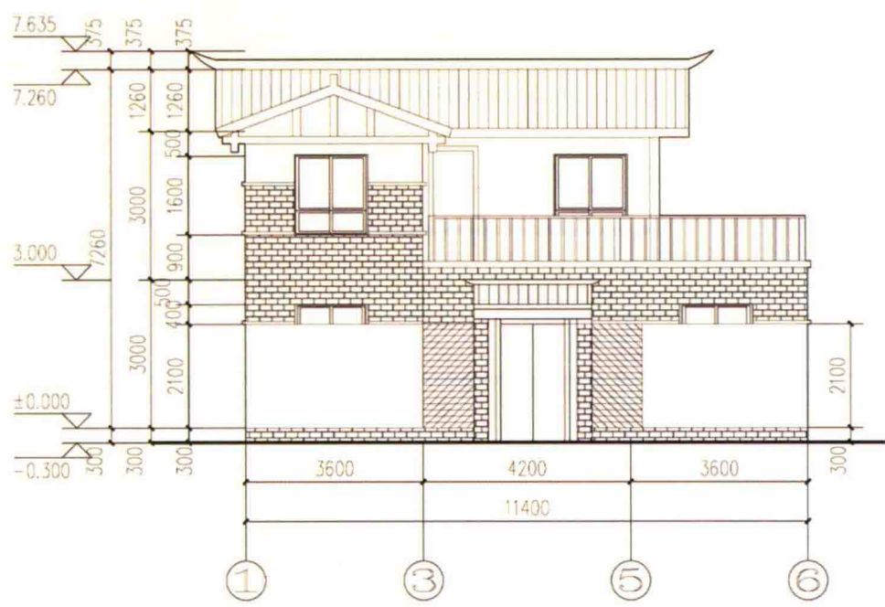
①-⑥立面图
