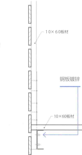
两侧截面图
