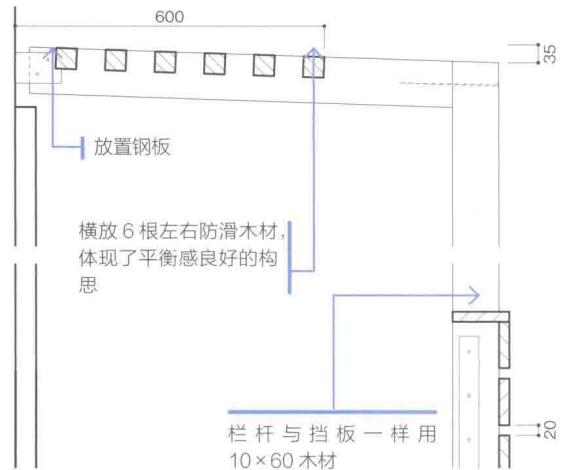
截面图
