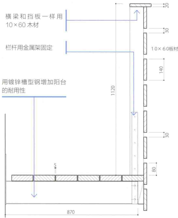
侧面截面图
