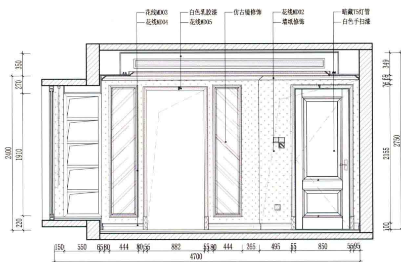
主卧立面图
