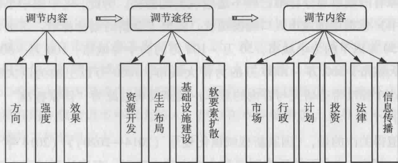
图 1-1 城市—区域系统的调节机能
